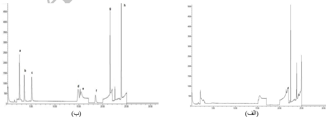
شکل 2. کروماتوگرام حاصل از استخراج توسط روش MAE-DLLME-GC-MS در حالت SIM. الف (بدون تزریق استاندارد) و نمونه ب (با تزریق استاندارد) از غلظت 40 \text{ ng g}^{-1} نیتروز آمین‌ها (a) (NDMA), (b) (NMEA), (c) (NDEA), (d) (NPYR), (e) (NPIP), (f) (NDBA), (g) biphenyl (IS), (h) N-(NDPheA)
