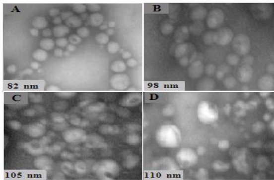
شکل 8: تصاویر لیپوزوم‌های حاوی DHA و EPA همراه ویتامین E در زمان صفر (A) با بزرگنمایی 80000 و پس از نگهداری به مدت 90 روز در دماهای 4°C (B)، 30°C (C) و 40°C (D) (به ترتیب با بزرگنمایی 40000، 80000 و 63000)
