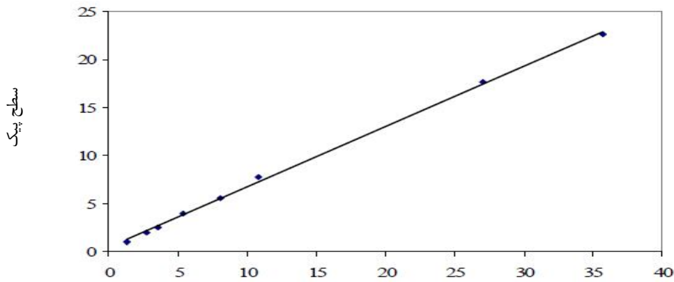
شکل 2. منحنی کالیبراسیون برای اندازه‌گیری کمی اولئوروپتین توسط دستگاه HPLC
