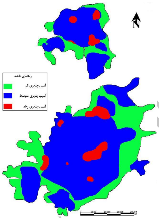
شکل ۴- نقشه قابلیت آسیب‌پذیری آبخوان دشت اسدآباد در مدل SI
