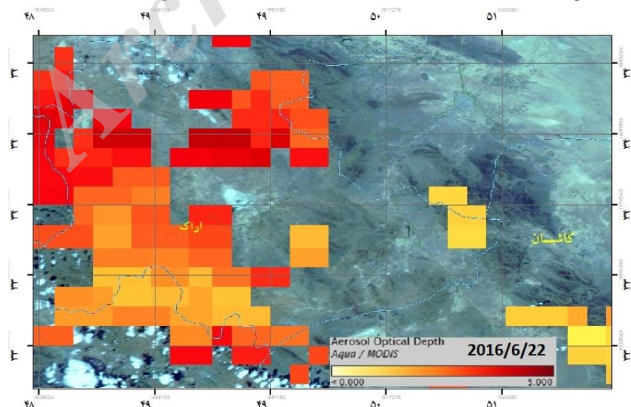
شکل ۵- تصویر گردوغبار بازسازی شده با استفاده از شاخص عمق اپتیکی تصاویر سنجنده MODIS در تاریخ ۲۰۱۶/۶/۲۲ Fig. 5- Image dust optical depth detection using MODIS images on June 22, 2016
