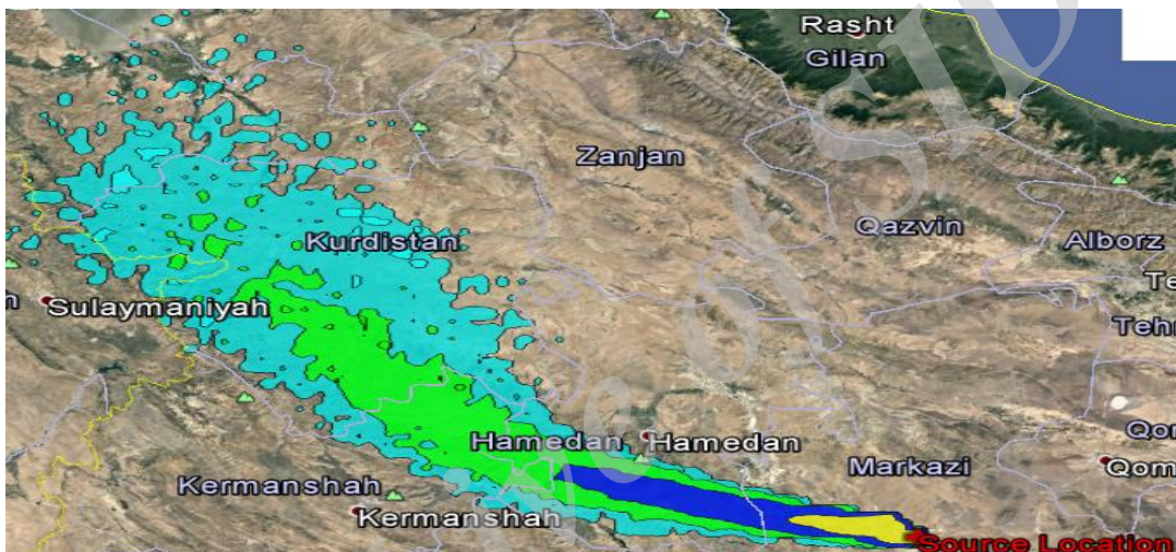
شکل ۴- مدل انتشار و مسیر رو به جلو انتقال گردوغبار از بستر و اراضی بیابانی حاشیه تالاب کویری میقان Fig. 4- Diffusion model and path forward transfer of dust from desert lands around the Meighan
