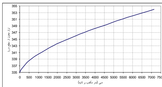
شکل 3 منحنی دبی-ارتفاع (دبی-اشل) مجموع سرریزهای سد دز
