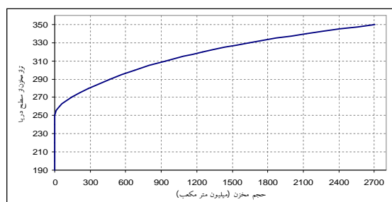
شکل 2 منحنی حجم - ارتفاع مخزن سد دز
