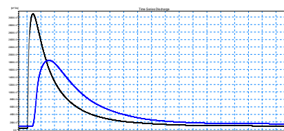
شکل 9 هیدروگراف سیلاب ناشی از شکست سد دز در محدوده رودخانه کارون (خط مشکی سد دز - خط آبی شهر دزفول - خط قرمز بند قیر) (خط مشکی ملاتانی - خط آبی شهر اهواز)
