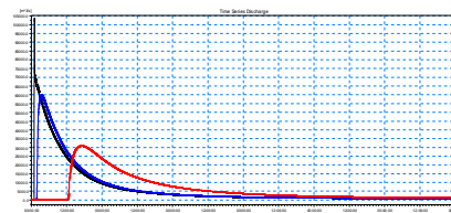
شکل 8 هیدروگراف سیلاب ناشی از شکست سد دز در محدوده رودخانه دز
