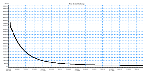
شکل 6 هیدروگراف ناشی از شکست سد دز
