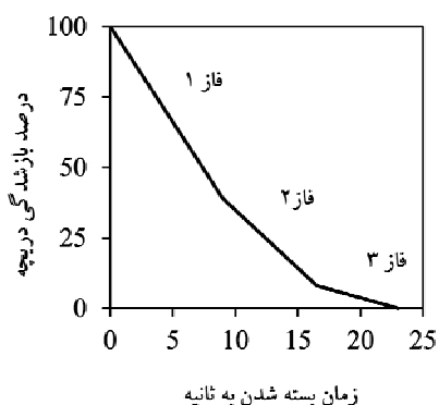
شکل 7 نتایج تحلیل هیدرولیکی دریچه (الگوی بسته شدن دریچه تونل آب بر سد و نیروگاه کارون 4)
