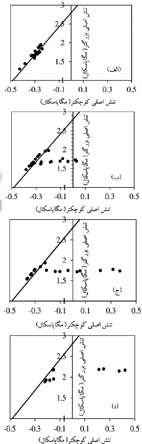
شکل 11 تنش‌های اصلی در المان‌های اطراف پوشش با افزایش روباره به میزان الف) 0.13H ، ب) 0.26H ، ج) 0.53H و د) 0.93H (زمان بسته شدن دریاچه در هر چهار حالت 14 ثانیه و هد استاتیکی آب 80 متر بوده است)
