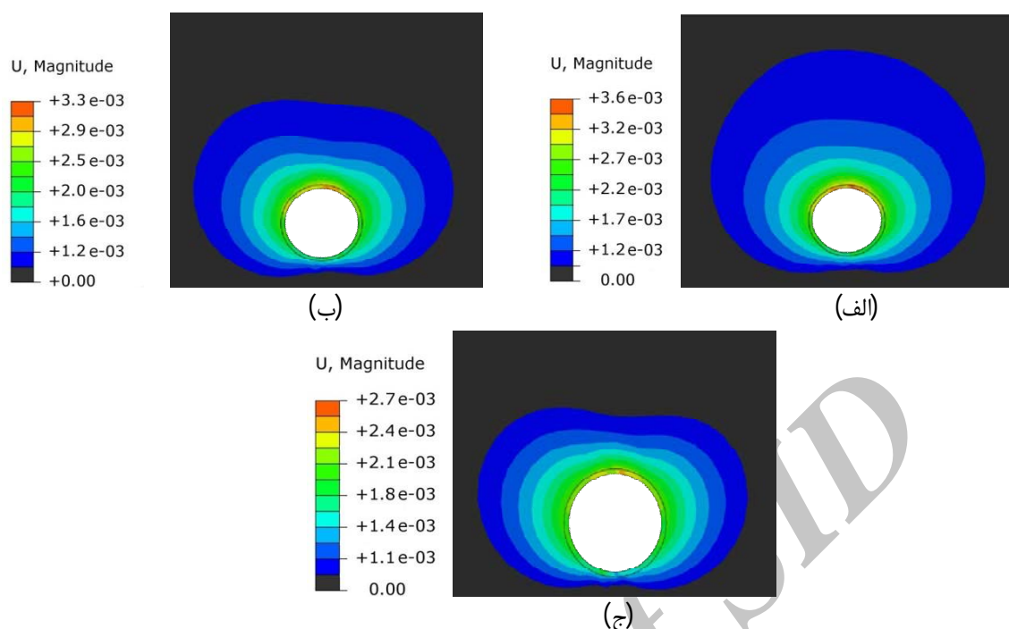
شکل 10 منحنی‌های هم‌تراز جابجایی در سنگ در لحظه (الف) - 14، (ب) - 18 و (ج) - 26 ثانیه برای تونل به قطر 3/6 متر و سرعت جریان درون تونل 6 متر بر ثانیه
