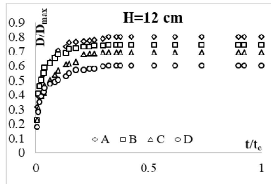
شکل 6 تغییرات زمانی حداکثر عمق آبشستگی با اضافه شدن رس و پلی اکریل آمید کاتیونی
