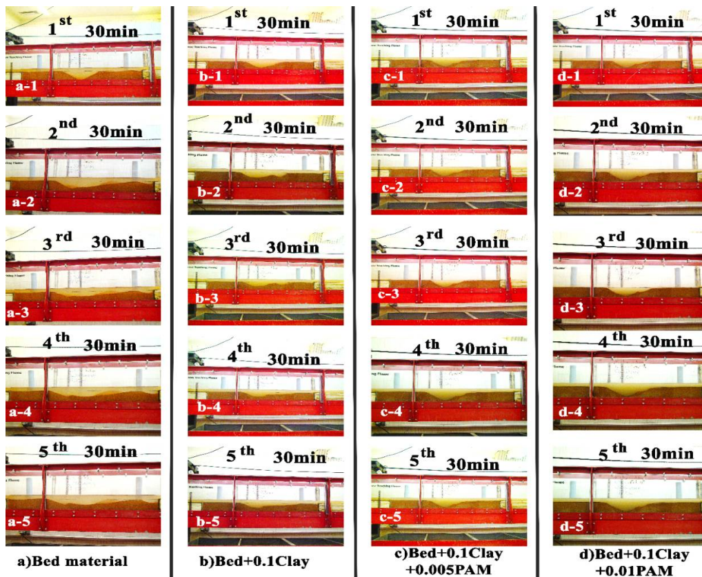
شکل 10 پروفیل های طولی آبشستگی
