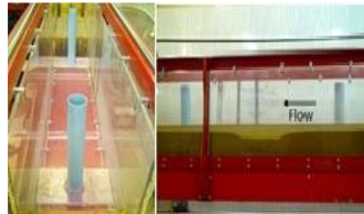
شکل 2 گودال، جهت جریان و قرار گیری پایه‌های پل در بستر متحرک
