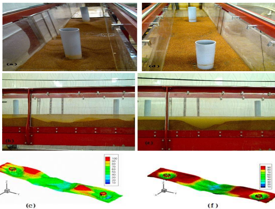
شکل 9 تغییرات طول و عمق آبشستگی اطراف پایه‌های پل و گودال‌های ایجاد شده - a, d - نما از بالا، e, b - نما از روبرو، c, f - نمای سه بعدی
