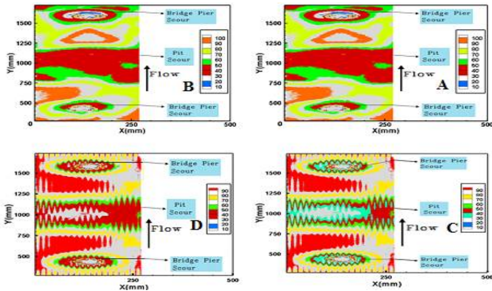
شکل 8 تغییرات دو بعدی عمق و طول آبشستگی در اطراف پایه‌های پل و گودال‌های ایجاد شده
