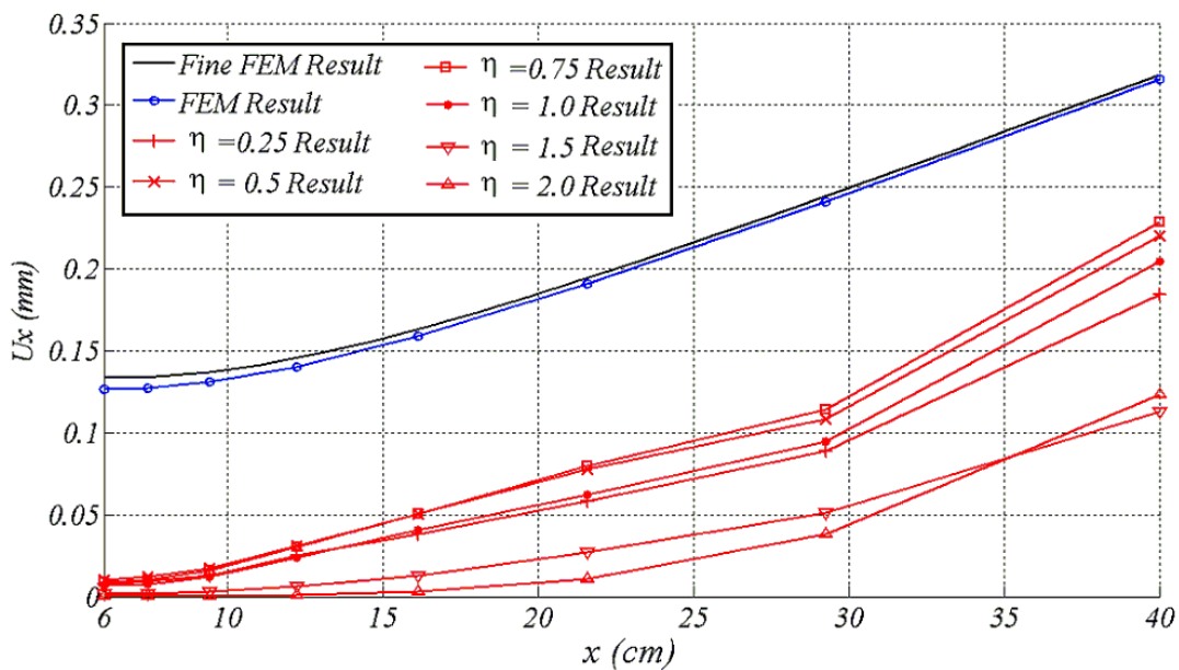
شکل 5 نمودار جابجائی در راستای افقی جهت گره های قرار گرفته بر روی خط y=0 برای مقادیر مختلف \eta برای تعداد همسایگی برابر با 4 گره
