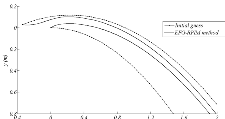
شکل 12 سطوح آزاد محاسبه شده بر اساس روش EFG-RPIM (سد شهپریار - مثال 3)
