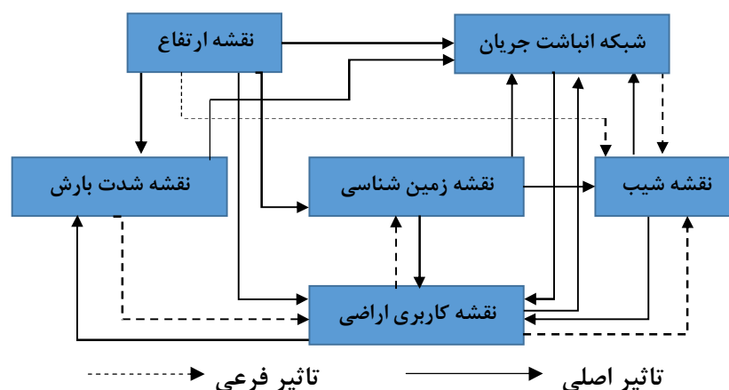
شکل 2 طرح شماتیک اندرکنش بین عوامل مؤثر در سیل خیزی حوضه
