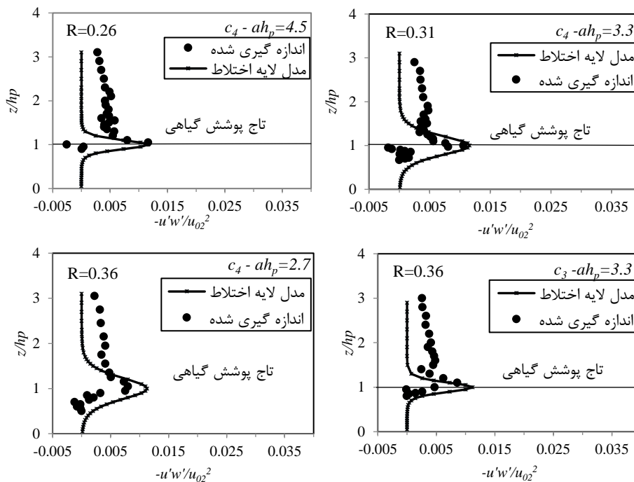
شکل ۱۴ مقایسه پروفیل تنش رینولدز برآورد شده از مدل لایه اختلاط با در نظر گرفتن جریان در حال توسعه با داده‌های اندازه‌گیری شده بر روی توده گیاهی مورد مطالعه در بازه انتخابی رودخانه بهشت‌آباد با سه تراکم مختلف
