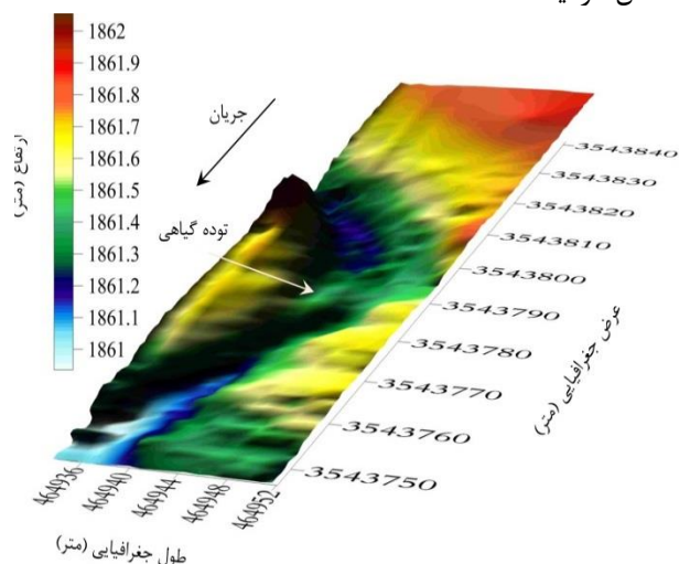
شکل ۲ توپوگرافی بازه انتخابی در رودخانه بهشت‌آباد
