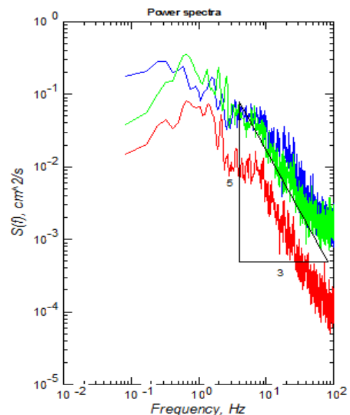
شکل ۵ ارزیابی صحت داده برداشت شده در زیر تاج پوشش گیاهی توسط ADV از طریق آنالیز اسپکترال
