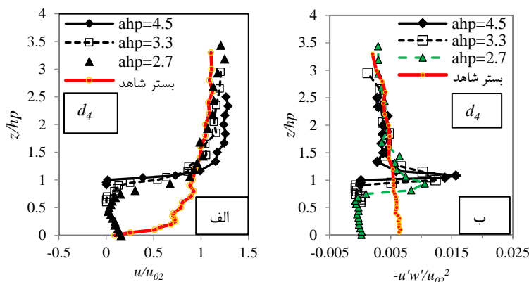
شکل ۷ الف) پروفیل سرعت افقی در موقعیت d_4 با سه تراکم مختلف و ب) پروفیل تنش رینولدز در موقعیت d_4 با سه تراکم مختلف
