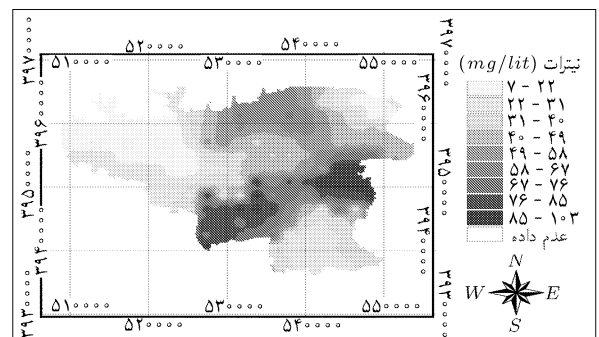
شکل ۵. غلظت نیترات برحسب میلی‌گرم بر لیتر نیتروژن با استفاده از مدل.
