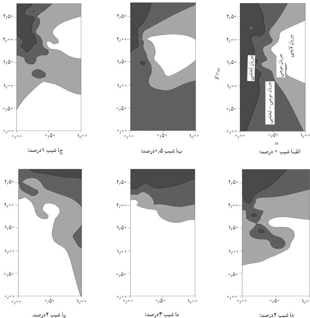
شکل ۷. نقشه‌ی الگوهای جریان برحسب عدد فرود و کسر فضای خالی در شیب‌های مختلف.
