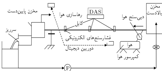
شکل ۴. شمای کلی بخش‌های مختلف مدل آزمایشگاهی.
