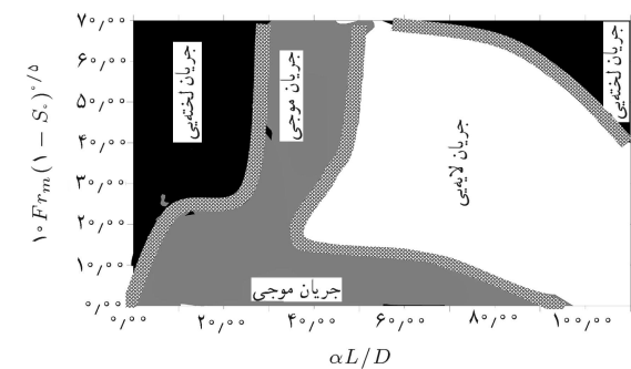
شکل ۹. نقشه‌ی الگوی جریان برحسب 10^5 Fr_m(1 - S_c)^{0.5} در مقابل \alpha L / D .
