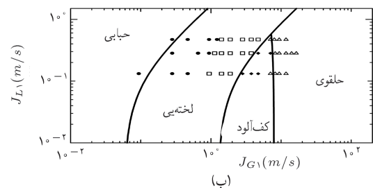
شکل ۳. الف) نقشه‌های الگوهای جریان دوفازی در مجرای افقی؛ [۱۷] ب) نقشه‌ی الگوهای جریان در اتصال T شکل. [۱۸]
