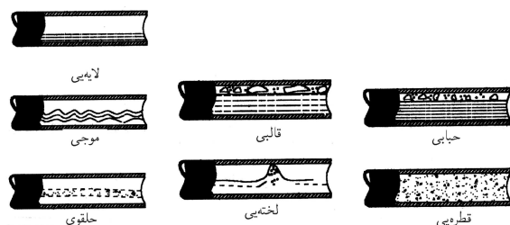
شکل ۱. الگوهای جریان دوفازی در مجاری افقی و شیب‌دار.
