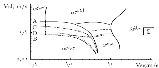
شکل ۲. نمودار تعیین الگوهای جریان دوفازی در خطوط لوله‌ی افقی نتایج؛ الف) Baker, ۱۹۷۵، ب) Mandhane, ۱۹۷۵ و ج) Federer, ۱۹۹۲.
