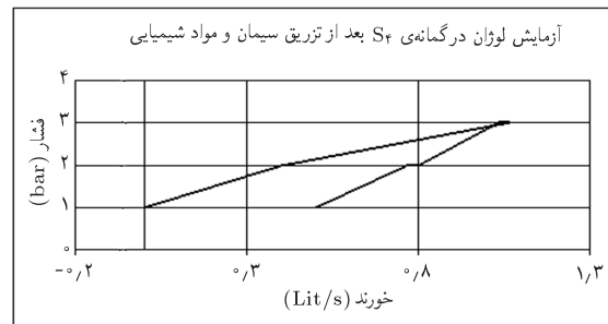
شکل ۹. نمودار فشار آزمایش و مقدار آب در گمانه‌ی S۴ بعد از تزریق سیمان و مواد شیمیایی. [۱۱]
