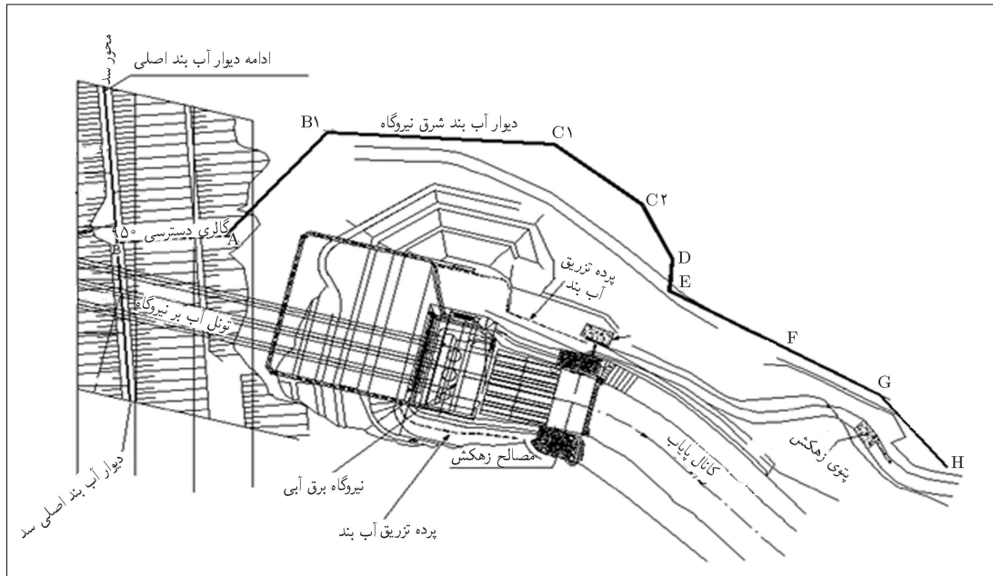
شکل ۶. پلان موقعیت سد کرخه، نیروگاه و دیوارهای آب بند.
