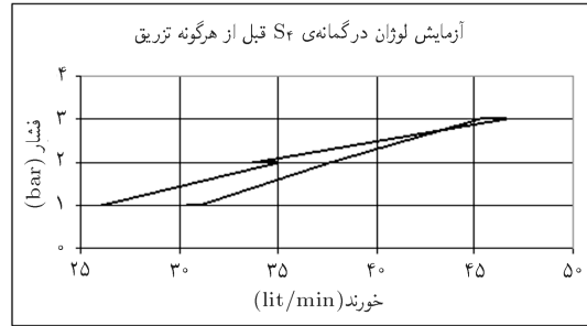
شکل ۸. نمودار فشار آزمایش و مقدار جذب آب در گمانه‌ی S۴ قبل از تزریق. [۱۱]
