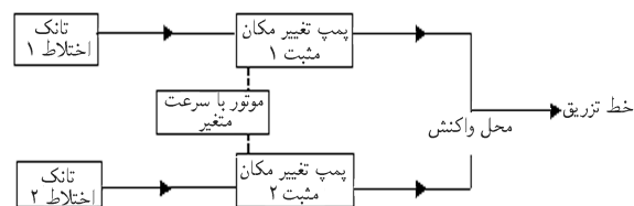
شکل ۲. نمودار شماتیک سیستم متشکل از دو پمپ و دو تانک مورد استفاده برای تهیه و تزریق دوغاب‌های شیمیایی.
