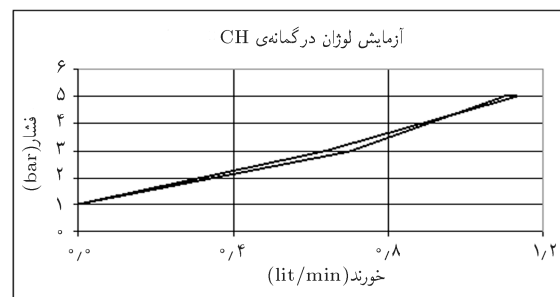
شکل ۱۳. نمودار فشار آزمایش و مقدار جذب آب در گمانه‌ی CH بعد از تزریق. [۱۱]
