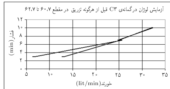
شکل ۱۲. نمودار فشار آزمایش و مقدار جذب آب در گمانه‌ی C۳ قبل از تزریق. [۱۱]
