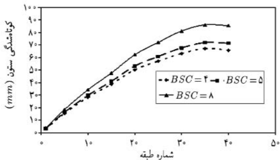
شکل ۱۵. مقادیر کوتاه‌شدگی ستون تحت تأثیر BSCهای مختلف.
