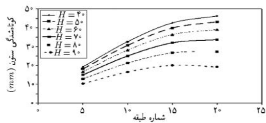
شکل ۷. مقادیر کوتاه شدگی ستون‌ها نسبت به تغییرات درصد رطوبت نسبی برای سازه‌ی ۲۰ طبقه.
