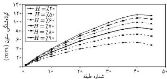
شکل ۱۰. مقادیر کوتاه شدگی ستون‌ها نسبت به تغییرات درصد رطوبت نسبی برای سازه‌ی ۴۵ طبقه.
