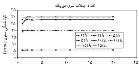
شکل ۱۱. مقایسه‌ی دوروش سری دیریکله و انتگرال‌گیری مستقیم در سازه‌ی ۱۵ طبقه.
