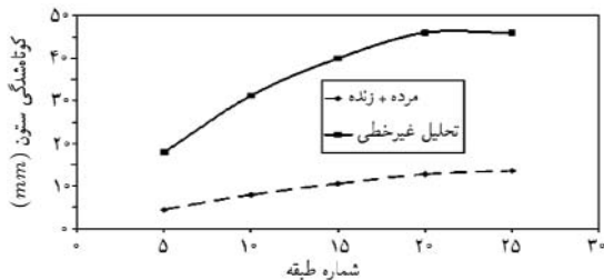
شکل ۱۴. مقادیر کوتاه‌شدگی ستون ناشی از آنالیزهای مختلف.
