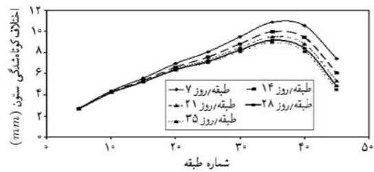
شکل ۶. مقادیر اختلاف کوتاه شدگی نسبت به تغییرات سرعت ساخت برای سازه‌ی ۴۵ طبقه.
