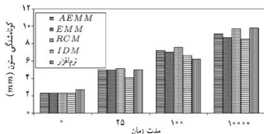
شکل ۱. نتایج مقایسه‌ی روش‌های IDM, RCM, EMM, AEMM با نتایج حاصل از نرم‌افزار.
