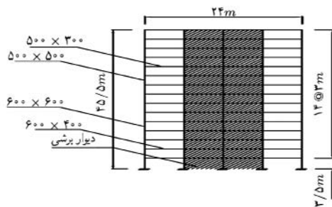
شکل ۲. مشخصات نمونه‌ی از قاب‌های مورد مطالعه.
