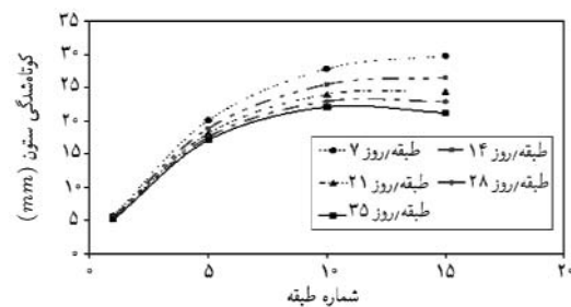
شکل ۳. مقادیر کوتاه‌شدگی ستون نسبت به سرعت ساخت‌های مختلف در سازه‌ی ۱۵ طبقه.
