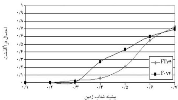
شکل ۳۰. مقایسه‌ی منحنی‌های شکنندگی تغییر شکل محوری قاب‌های FOV4 و FTV4 در سطح LS.
