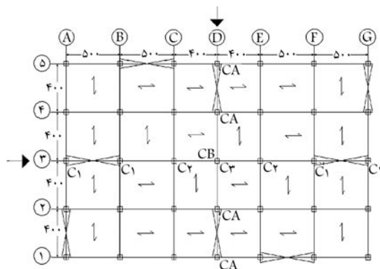
شکل ۱. پلان ساختمان‌های ۳، ۵ و ۷ طبقه برای قاب‌های ۴ و ۶ دهانه در جانمایی جدا از هم.
