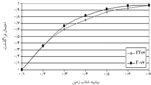
شکل ۲۹. مقایسه‌ی منحنی‌های شکنندگی تغییر شکل محوری قاب‌های FOV4 و FTV4 در سطح IO.
