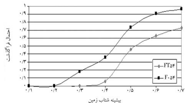
شکل ۲۴. مقایسه‌ی منحنی‌های شکنندگی تغییر شکل محوری قاب‌های FT۵۴ و FO۵۴ در سطح LS.
