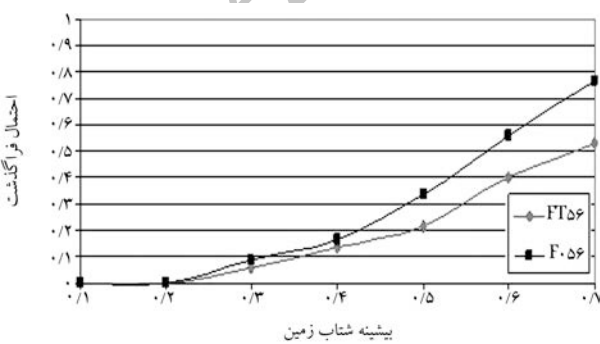
شکل ۲۸. مقایسه‌ی منحنی‌های شکنندگی تغییر شکل محوری قاب‌های FT۵۶ و FO۵۶ در سطح CP.
