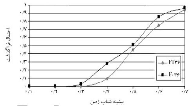
شکل ۲۲. مقایسه‌ی منحنی‌های شکنندگی تغییر شکل محوری قاب‌های FT۳۶ و FO۳۶ در سطح CP.
