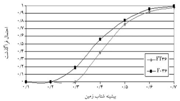
شکل ۲۱. مقایسه‌ی منحنی‌های شکنندگی تغییر شکل محوری قاب‌های FT۳۶ و FO۳۶ در سطح LS.
