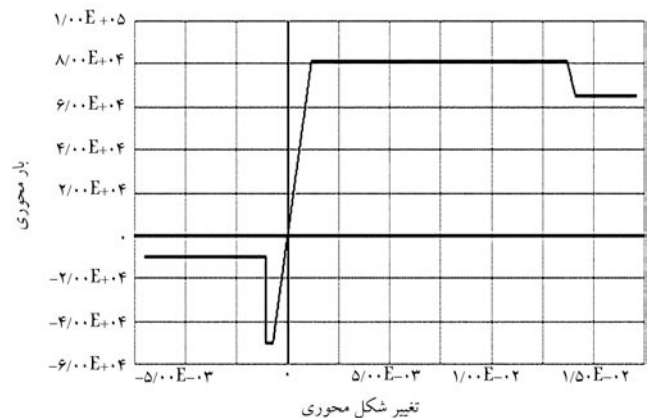
شکل ۶. نمونه‌ی از مدل رفتاری مهاربند 2UNP120 معرفی شده به برنامه ۳D-PERFORM. [۶]
