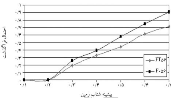
شکل ۲۷. مقایسه‌ی منحنی‌های شکنندگی تغییر شکل محوری قاب‌های FT۵۶ و FO۵۶ در سطح LS.
