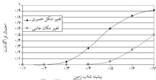
شکل ۱۵. مقایسه‌ی منحنی‌های شکنندگی تغییر مکان بین طبقه‌ی بی و تغییر شکل محوری سازه‌های ۳ طبقه در سطح LS.
