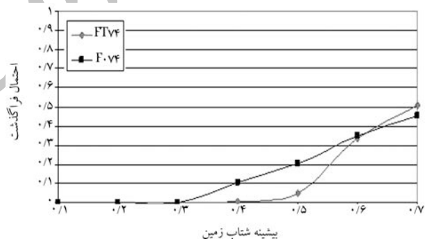
شکل ۳۱. مقایسه‌ی منحنی‌های شکنندگی تغییر شکل محوری قاب‌های FOV4 و FTV4 در سطح CP.
