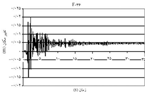
شکل ۷. تاریخچه‌ی زمانی تغییر مکان تراز بام برای قاب FO۳۶ با جانمایی جدا تحت اثر شتاب‌نگاشت سان‌فرناندو در سطح ۰٫۴g.
