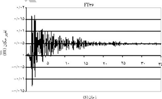
شکل ۸. تاریخچه‌ی زمانی تغییر مکان تراز بام برای قاب FT۳۶ با جانمایی به هم چسبیده برای شتاب‌نگاشت سان‌فرناندو در سطح ۰٫۴g.
