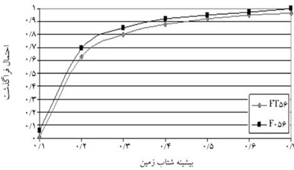
شکل ۲۶. مقایسه‌ی منحنی‌های شکنندگی تغییر شکل محوری قاب‌های FT۵۶ و FO۵۶ در سطح IO.
