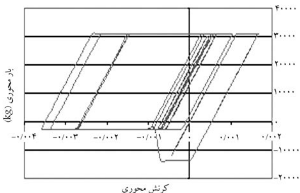
شکل ۹. منحنی تغییرات نیروی محوری نسبت به کرنش محوری برای مهاربند طبقه‌ی اول از قاب BT۳۶ برای شتاب‌نگاشت لوماپریتا در سطح ۰٫۴g.
