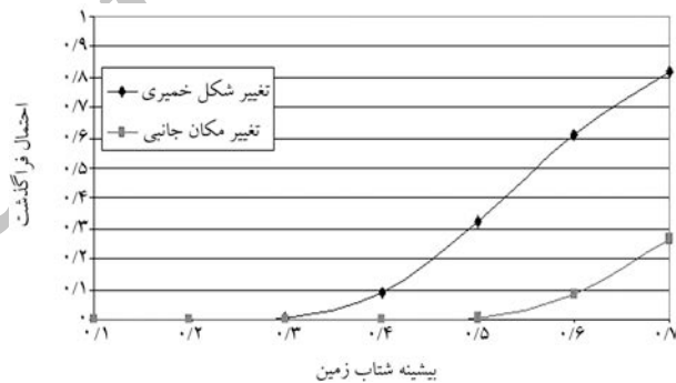
شکل ۱۶. مقایسه‌ی منحنی‌های شکنندگی تغییر مکان بین طبقه‌ی بی و تغییر شکل محوری سازه‌های ۳ طبقه در سطح CP.
