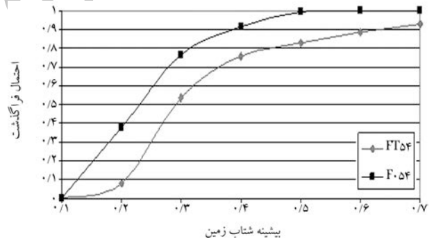
شکل ۲۳. مقایسه‌ی منحنی‌های شکنندگی تغییر شکل محوری قاب‌های FT۵۴ و FO۵۴ در سطح IO.
