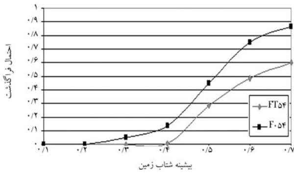
شکل ۲۵. مقایسه‌ی منحنی‌های شکنندگی تغییر شکل محوری قاب‌های FT۵۴ و FO۵۴ در سطح CP.
