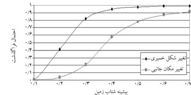
شکل ۱۴. مقایسه‌ی منحنی‌های شکنندگی تغییر مکان بین طبقه‌ی بی و تغییر شکل محوری سازه‌های ۳ طبقه در سطح IO.
