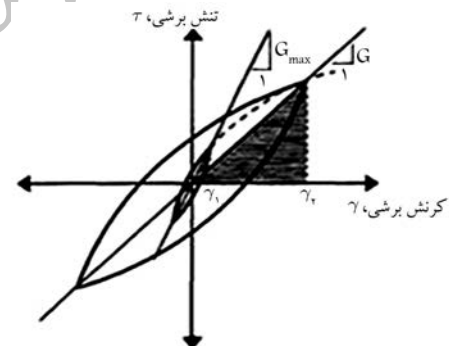
شکل ۲. مدول برشی تاثرناخت (Gmax) و مدول برشی سکانت (Gsec).
