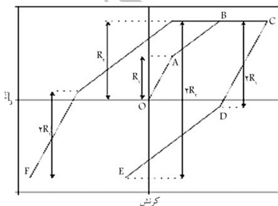
شکل ۱۶. متحنی تنش-کرنش خاک براساس مدل ایوان و مرز.
