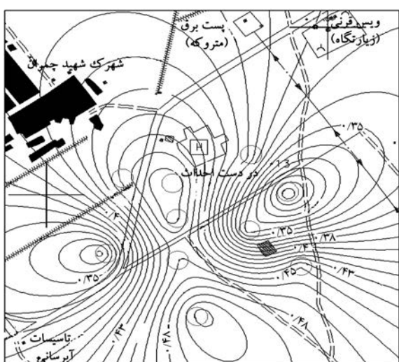
شکل ۱۲. نقشه‌ی هم‌تراز بیشینه تابع بزرگ‌نمایی؛ بیشینه شتاب سنگ بستر g °/۲.
