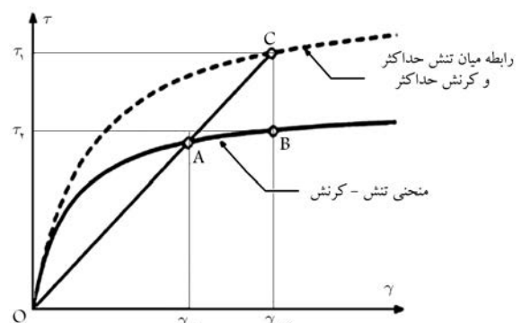
شکل ۳. نمودار شماتیک نشان‌دهنده‌ی بیش تخمینی تنش برشی در روش خطی معادل.
