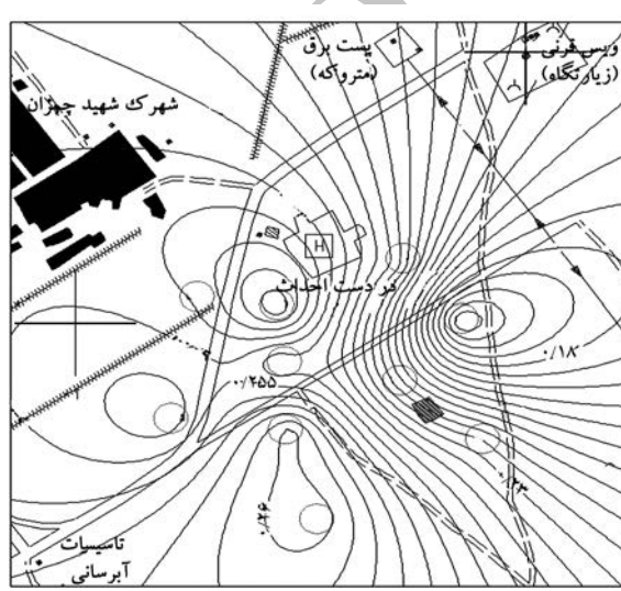
شکل ۹. نقشه‌ی هم‌تراز بیشینه‌ی شتاب سطح زمین (g)؛ بیشینه شتاب سنگ بستر g °/۲.
