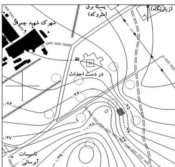
شکل ۱۱. نقشه‌ی هم‌تراز بیشینه تابع بزرگ‌نمایی؛ بیشینه شتاب سنگ بستر g °/۳۵.
