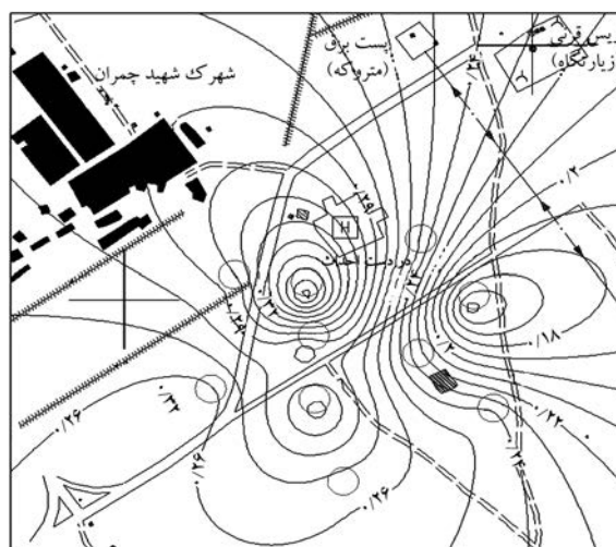
شکل ۱۰. نقشه‌ی هم‌تراز بیشینه‌ی شتاب سطح زمین (g)؛ بیشینه شتاب سنگ بستر g °/۳۵.
