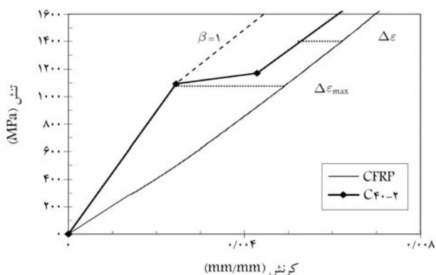
شکل ۱۲. معرفی \Delta \varepsilon ، \Delta \varepsilon_{max} و \beta .
