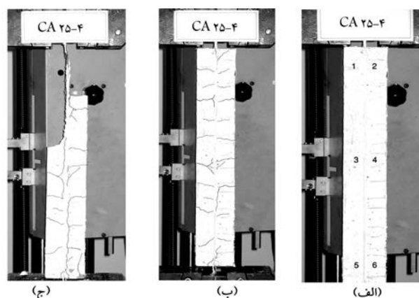
شکل ۴. مراحل بارگذاری نمونه‌ی CA۲۵-۴.
