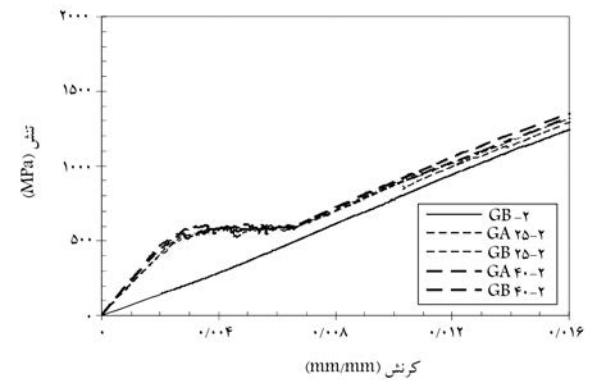
شکل ۷. منحنی تنش - کرنش نمونه‌های دارای دو لایه GFRP.
