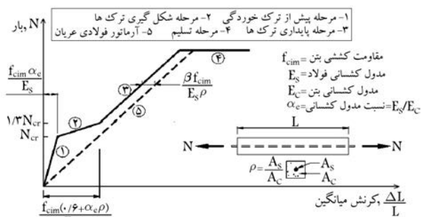
شکل ۱. رابطه‌ی بار - کرنش بتن مسلح تحت کشش. [۷]
