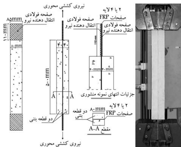
شکل ۲. جزئیات و مشخصات نمونه‌های بتنی و نمونه‌ی بتنی قرارگرفته در فک‌های دستگاه کشش.
