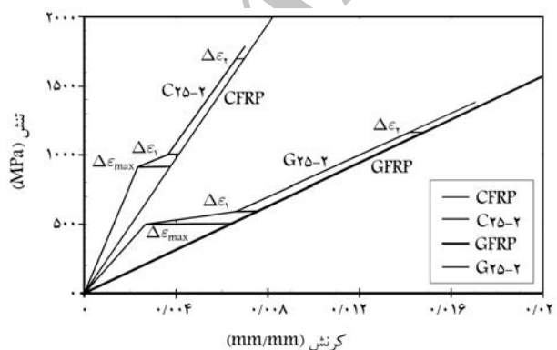
شکل ۱۳. میزان اثر سخت‌کنندگی کششی نمونه‌های C25-2 و G25-2 در مرحله ترک‌خوردگی پایدار.
