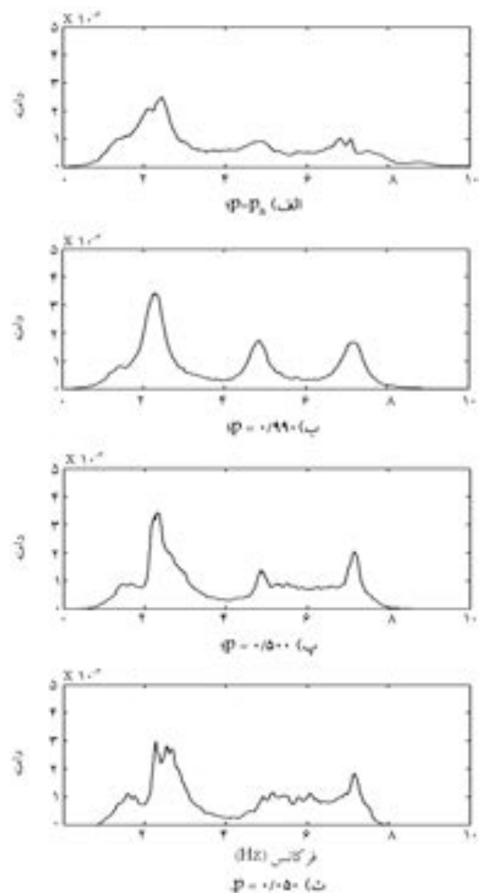
شکل ۹. طیف حاشیه‌ی میانگین حاصل از روش ارتقاء یافته.
