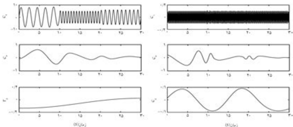
شکل ۵. توابع مودی ذاتی متناظر با سیگنال g(t) .
