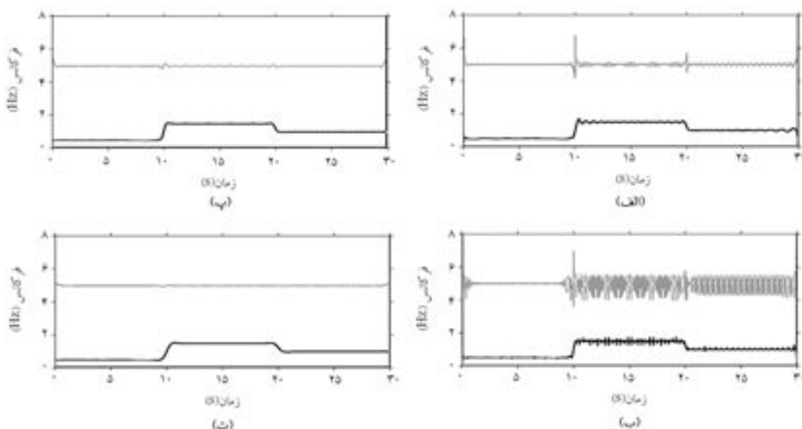
شکل ۶. طیف‌های هیلبرت - هوآنگ کلاسیک و هیلبرت - هوآنگ ارتقاء یافته متناظر با دو تابع مودی ذاتی اول g(t) .
