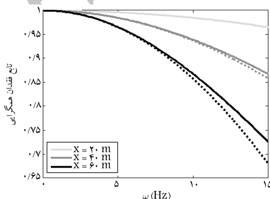
شکل ۹. بررسی تغییرات تابع فقدان همگرایی دقیق (خط) و تقریبی (خط چین)، در مقابل بسامد به ازاء مقادیر مختلف x = 20, 40, 60 m و \lambda_x / V_S = 0.0001 .
