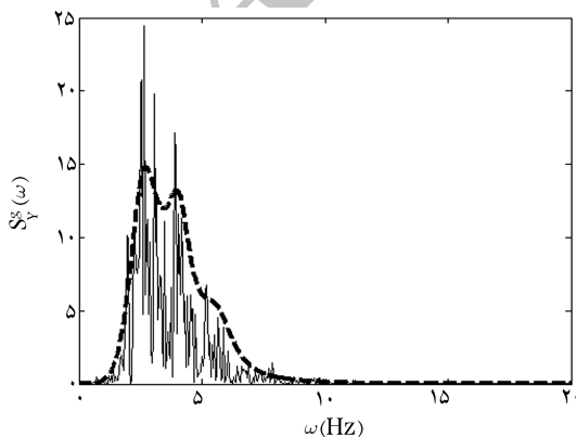
شکل ۲. چگالی طیفی شتاب مؤلفه‌ی افقی زلزله در راستای محور y.
