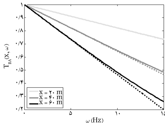
شکل ۱۰. بررسی تغییرات T_{BA}(\omega) دقیق (خط) و تقریبی (خط چین)، در مقابل بسامد به ازاء مقادیر مختلف x = 20, 40, 60 m و \lambda_x / V_S = 0.0001 .
