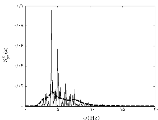
شکل ۶. چگالی طیفی شتاب مؤلفه‌ی پیچشی زلزله.
