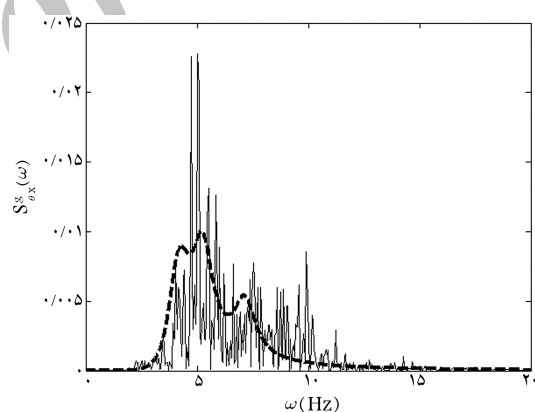
شکل ۴. چگالی طیفی شتاب مؤلفه‌ی گهواره‌یی زلزله در راستای محور x .
