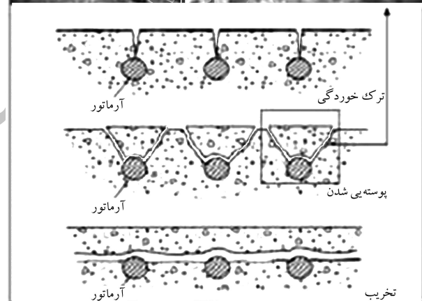
شکل ۸. ایجاد ترک به‌علت خوردگی آرماتورها.
