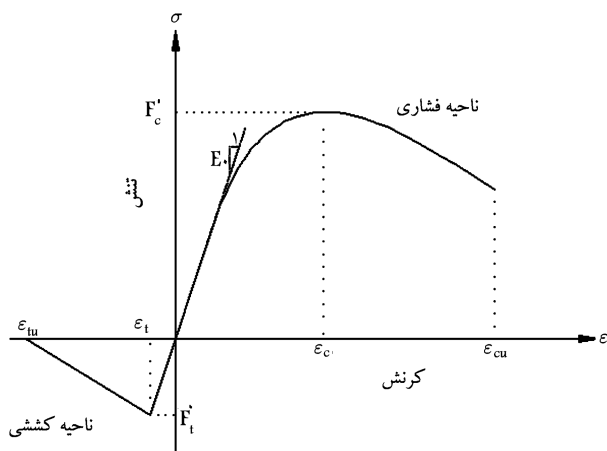
شکل ۱. منحنی تنش-کرنش بتن در کشش و فشار.
