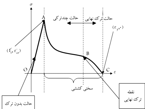
شکل ۹. نمایش شماتیک منحنی سخت‌شوندگی کششی.
