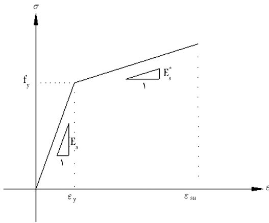
شکل ۲. منحنی تنش- کرنش فولاد در کشش و فشار.
