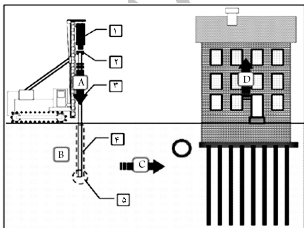
شکل ۲. انتقال ارتعاشات از چکش تا سازه‌های مجاور از طریق خاک. [۱]
