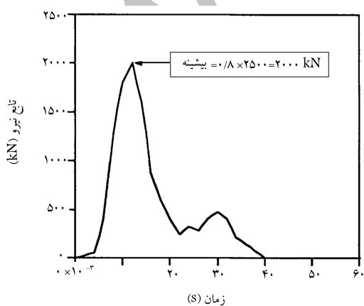
شکل ۳. نمودار نیرو - زمان اعمال‌شده بر سر شمع. [۱۵]
