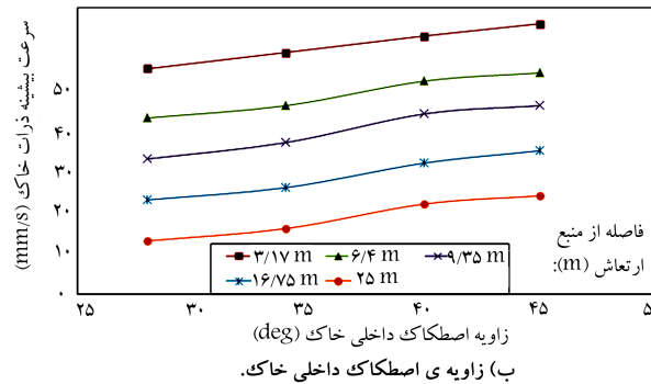
شکل ۸. مقادیر سرعت بیشینه‌ی ذرات در فواصل مختلف از شمع.
