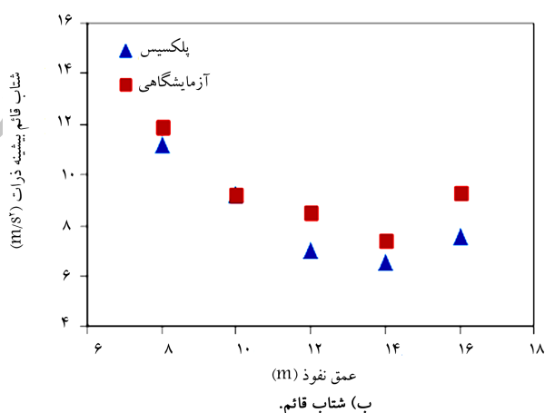
شکل ۴. مقادیر بیشینه شتاب ذرات خاک در فاصله‌ی ۳ متری از محل کوبش در سطح زمین.
