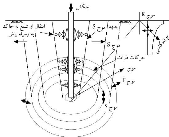
شکل ۱. امواج ساطع شده در اثر فرایند شمع‌کوبی.
