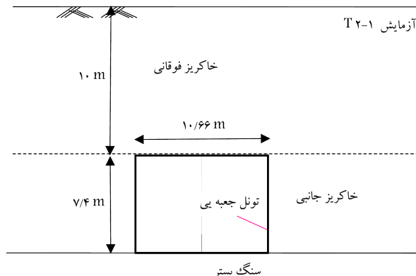
شکل ۲. آزمایش T۲-۱ در مقیاس پروتوتایپ.
