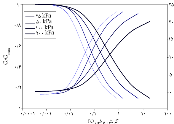
شکل ۳. تغییرات منحنی G/G_{max} و نسبت میرایی در برابر کرنش برشی ماسه‌ی مورد آزمایش.
