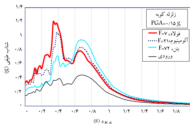
شکل ۱۵. طیف پاسخ شتاب در سطح زمین برای مصالح پوشش با ضریب انعطاف‌پذیری متفاوت - زلزله‌ی کوبه PGA = 0.15g .
