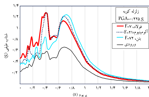
شکل ۱۶. طیف پاسخ شتاب در سطح زمین برای مصالح پوشش با ضریب انعطاف‌پذیری متفاوت - زلزله‌ی کوبه PGA = 0.225g .
