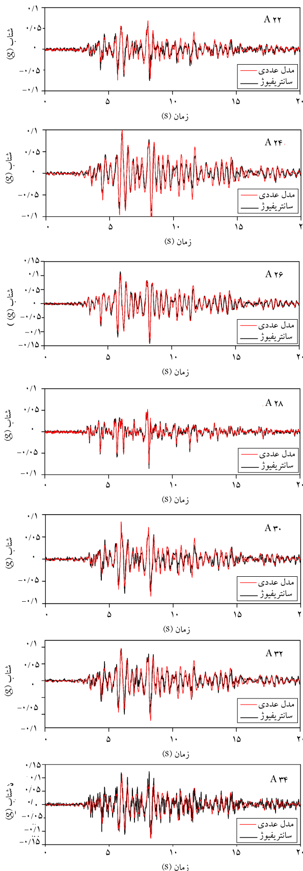
شکل ۱۰. نتایج شبیه‌سازی عددی آزمایش ۱-T۲: زلزله‌ی کوبه با 0.088g PGA =
