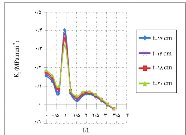
شکل ۹. منحنی تغییرات ضریب شدت تنش مود I ( K_I ) با فاصله‌ی خودرو از ترک ( l/L ) و برای ضخامت‌های مختلف رویه‌ی آسفالتی.
