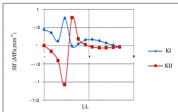
شکل ۱۳. مقایسه ی مقادیر K_I با K_{II} برای فواصل مختلف خودرو از محل ترک.
