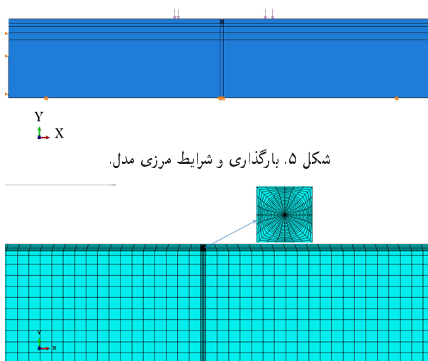
شکل ۶. مدل المان محدود روسازی آسفالتی تحت بارگذاری ناشی از عبور چرخ‌ها و نمای نزدیکی از المان‌های اطراف ترک.
