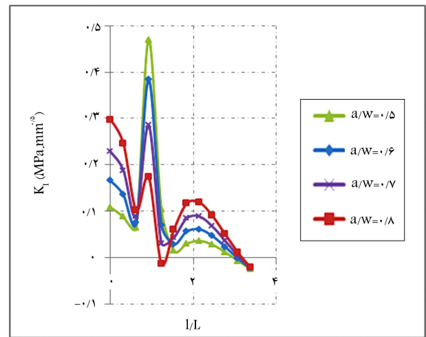
شکل ۸. منحنی تغییرات ضریب شدت تنش مود I ( K_I ) با فاصله‌ی خودرو از ترک ( l/L ) و برای طول‌های مختلف ترک ( a/w ).
