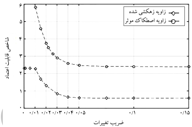
شکل ۷. شاخص قابلیت اعتماد در برابر ضریب تغییرات دو پارامتر برای شمع بتنی در خاک‌های غیرچسبنده.
