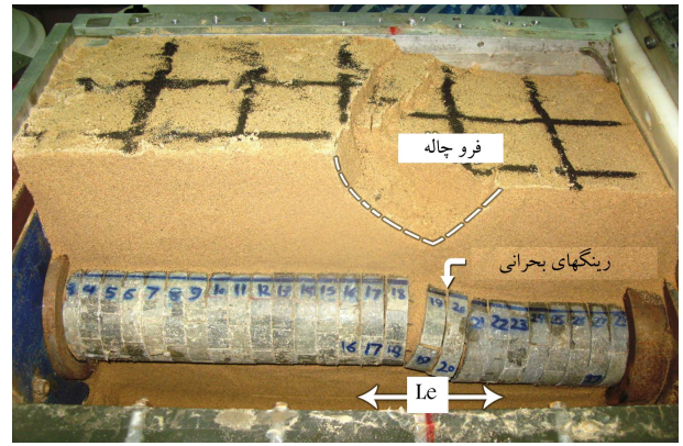
شکل ۱۳. تغییر شکل طولی تونل و فروچاله در سطح زمین در گسلش عادی.
