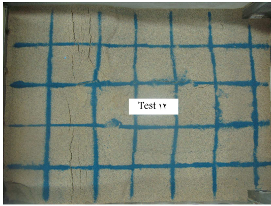
شکل ۱۵. ایجاد ترک در سطح زمین در سمت فرادیواره در اثر گسلش معکوس.
