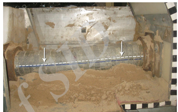
شکل ۱۴. تغییر شکل طولی تونل قطعه‌ی بی در گسلش معکوس.
