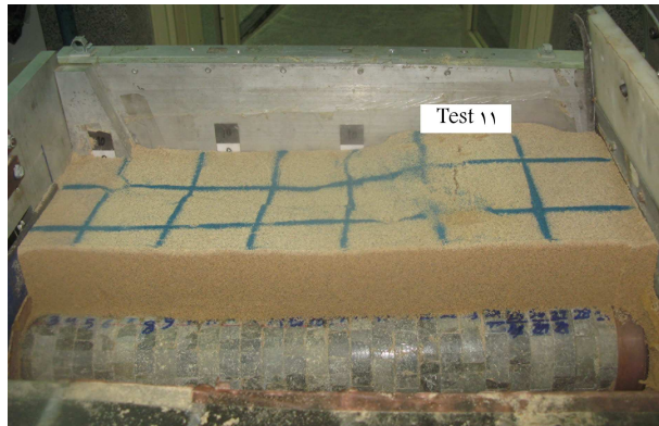
شکل ۱۶. تصویر سطح زمین در گسلش معکوس - روباره ۰/۷۵D.
