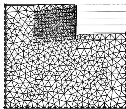
جابجایی کل 77/96 \times 10^{-3} \text{ m} (بزرگنمایی ۲۰ برابر)
