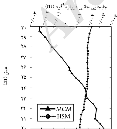
ب) تغییر شکل دیواره ی گود.
