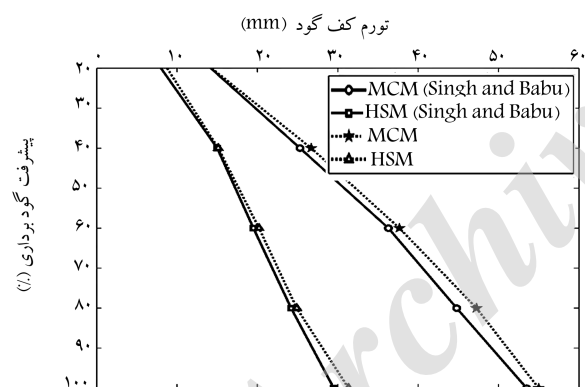
الف) تغییر شکل کف گود؛
