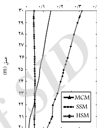
(ب) تغییر شکل دیواره ی گود.
