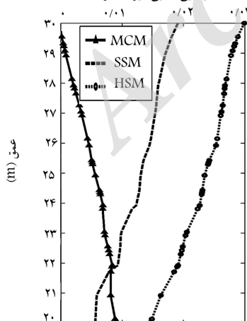
(ب) تغییر شکل دیواره ی گود.
