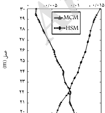
ب) تغییر شکل دیواره ی گود.
