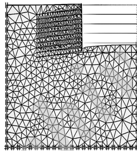
جایجایی کل 80/86 \times 10^{-3} m
