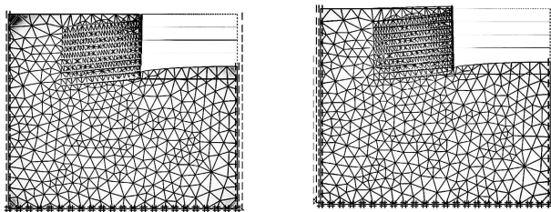
جابجایی کل 96/58 \times 10^{-3} \text{ m} (بزرگنمایی ۲۰ برابر) (ب) مدل سازی با مدل رفتاری خاک نرم شونده؛
