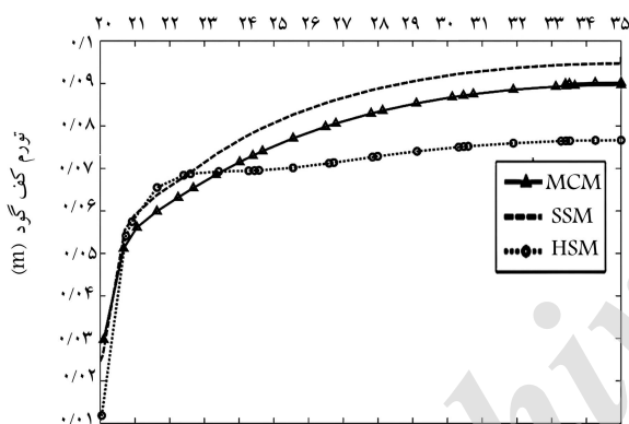
(الف) تغییر شکل کف گود؛
