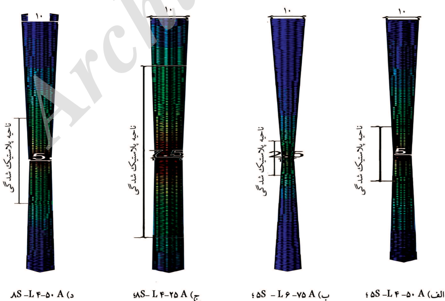
شکل ۱۲. نسبت تنش موجود به تنش مجاز در حالت خطی برای ۴ مدل از مهاربندهای کماتش تاب.
