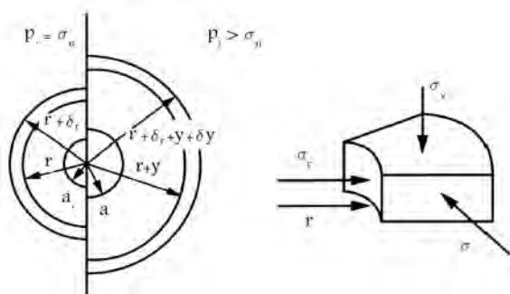
شکل ۱. انبساط حفره.
