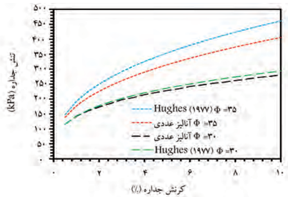
شکل ۱۴. مقایسه‌ی آنالیز عددی و روش هوگه (۱۹۷۷).
