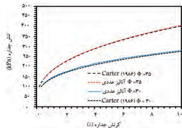
شکل ۱۳. مقایسه‌ی آنالیز عددی و روش کارتر (۱۹۸۶).
