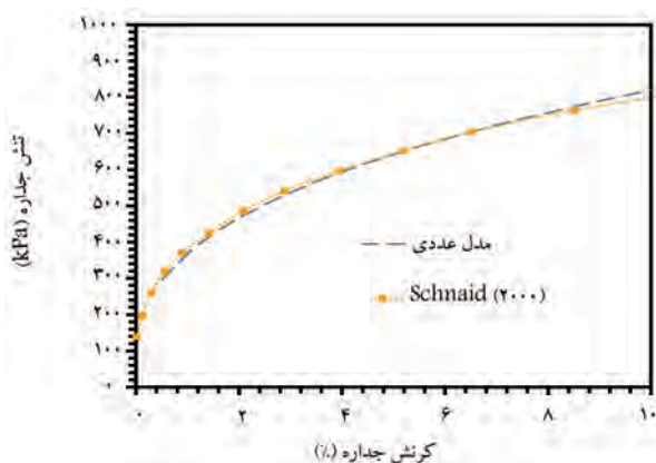
شکل ۱۲. مقایسه‌ی مدل عددی با مدل ایشنید (۲۰۰۰).
