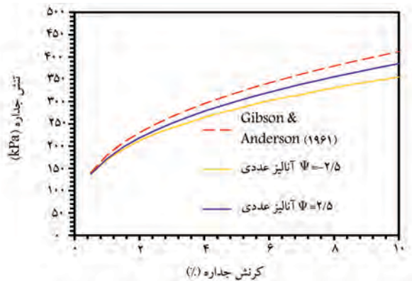
شکل ۱۵. مقایسه‌ی آنالیز عددی و روش گیبسون و آندرسون (۱۹۶۱).
