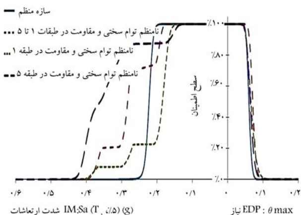
شکل ۱۰. نمودار تغییرات سطح اطمینان عدم تجاوز از سطح عملکردی CP در برابر تقاضای جابجایی و شدت ارتعاشات برای مدل‌های نامنظم توام سختی و مقاومتی.
