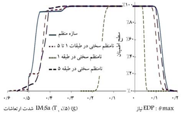
شکل ۱۲. نمودار تغییرات سطح اطمینان عدم تجاوز از سطح عملکرد GI در برابر تقاضای جابجایی و شدت ارتعاشات برای مدل‌های نامنظم سختی.
