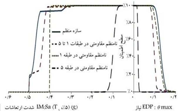
شکل ۱۳. نمودار تغییرات سطح اطمینان عدم تجاوز از سطح عملکرد GI در برابر تقاضای جابجایی و شدت ارتعاشات برای مدل‌های نامنظم مقاومتی.
