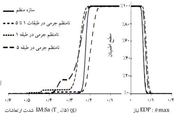
شکل ۷. نمودار تغییرات سطح اطمینان عدم تجاوز از سطح عملکردی CP در برابر تقاضای جابجایی و شدت ارتعاشات برای مدل‌های نامنظم جرمی.
