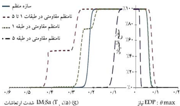
شکل ۹. نمودار تغییرات سطح اطمینان عدم تجاوز از سطح عملکردی CP در برابر تقاضای جابجایی و شدت ارتعاشات برای مدل‌های نامنظم مقاومتی.
