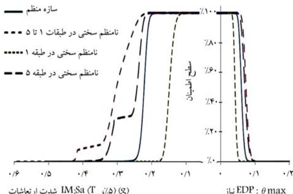
شکل ۸. نمودار تغییرات سطح اطمینان عدم تجاوز از سطح عملکردی CP در برابر تقاضای جابجایی و شدت ارتعاشات برای مدل‌های نامنظم سختی.
