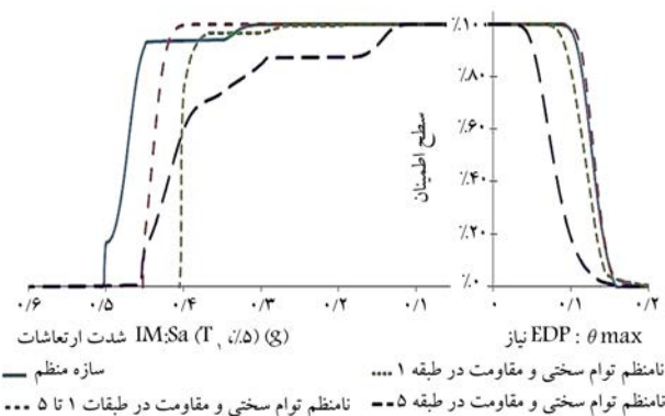
شکل ۱۴. نمودار تغییرات سطح اطمینان عدم تجاوز از سطح عملکرد GI در برابر تقاضای جابجایی و شدت ارتعاشات برای مدل‌های نامنظم توأم سختی و مقاومت.
