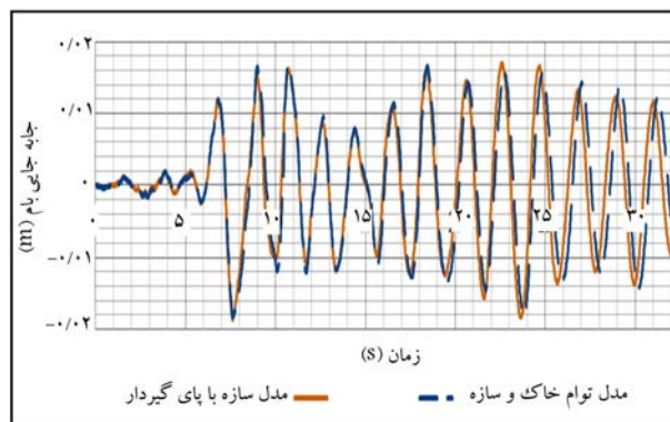
شکل ۴. مقایسه‌ی پاسخ بام سازه به منظور صحت‌سنجی مدل تحلیلی.
