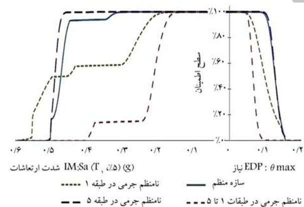
شکل ۱۱. نمودار تغییرات سطح اطمینان عدم تجاوز از سطح عملکردی GI در برابر تقاضای جابجایی و شدت ارتعاشات برای مدل‌های نامنظم جرمی.
