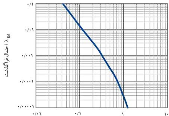
شکل ۶. منحنی خطر سایت.
