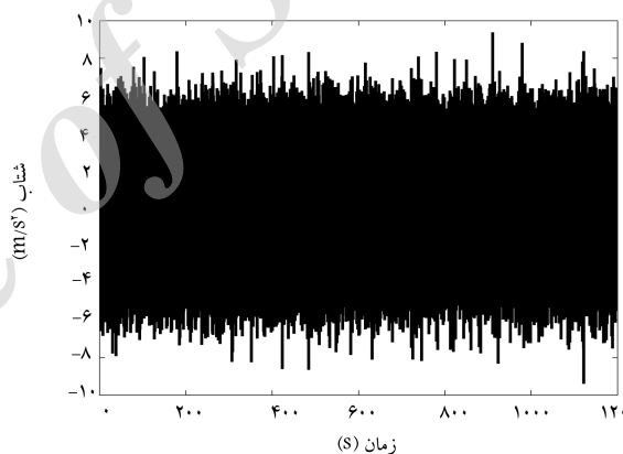
شکل ۱۶. سیگنال شتاب خروجی نایستای راستای قائم متناظر با نقطه‌ی ۱۱.
