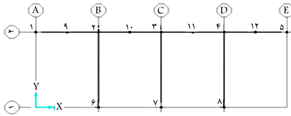
شکل ۱۴. قاب دوبعدی مدل شده در نرم‌افزار SAP۲۰۰۰.
