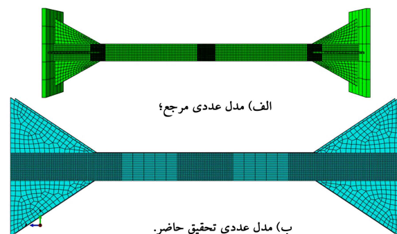
شکل ۶. نمایشی از تیر مدل شده.
