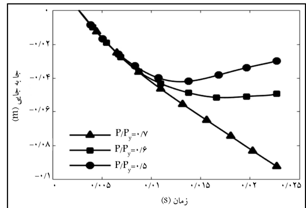
شکل ۱۳. مقدار جابه‌جایی عرضی ستون فولادی تحت بارگذاری‌های مختلف فشاری محوری.
