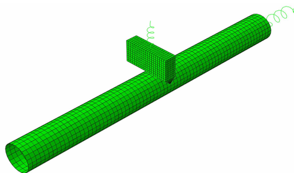
شکل ۳. شبیه‌سازی عددی پرتابه و ستون فولادی جهت صحت‌سنجی با مدل آزمایشگاهی.
