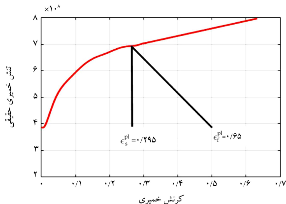
شکل ۵. خصوصیات مربوط به فولاد S۳۵۵ مورد استفاده در این پژوهش. [۲۲]
