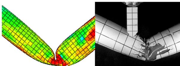
شکل ۱۴. تغییر شکل عرضی ستون فولادی تحت ضربه با سرعت ۷ متر بر ثانیه و پیش بار (P/P_y = 0.7) . [۱]
