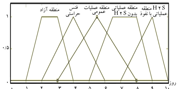
نمودارهای توابع عضویت فازی جهت تعیین زمان لازم برای تهیه 200 \text{ m}^3 بتن با رویکرد تأثیر ضوابط HSE (day)
