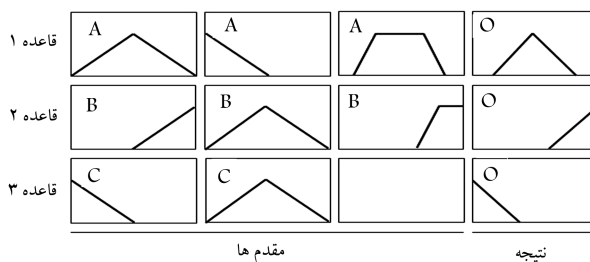
شکل ۳. مرحله‌ی ورودی و فازی‌سازی مثال موردی.
