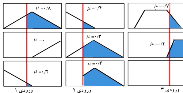
شکل ۴. دیاگرام استنتاج فازی مثال موردی.
