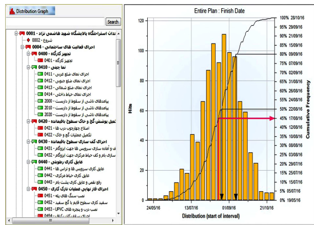
شکل ۲۰. خروجی گرافیکی آنالیز برنامه ی زمان بندی بر مبنای مدل پیشنهادی پژوهش.
