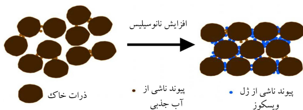
شکل ۸. اثر نانوسیلیس در فاصله ی بین ذرات رس. [۲۸]
