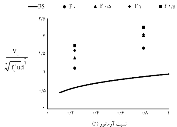
شکل ۱۱. اثر نسبت آرماتور خمشی و الیاف در ظرفیت برش پانچینگ آیین‌نامه‌ی BS.
