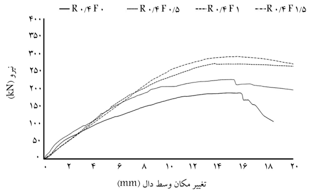
شکل ۶. نمودار بار - تغییر مکان نمونه‌های با نسبت آرماتور ۰٫۴٪.
