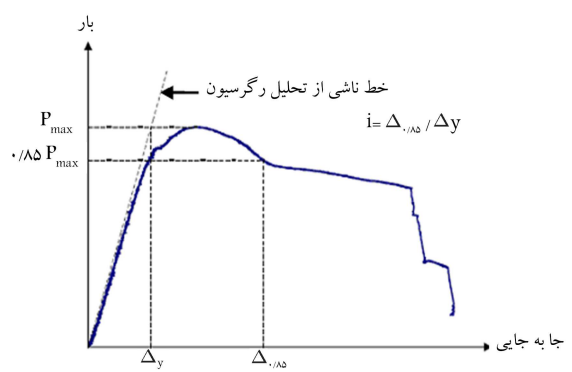
شکل ۹. چگونگی محاسبه‌ی شاخص شکل‌پذیری.
