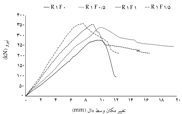
شکل ۷. نمودار بار - تغییر مکان نمونه‌های با نسبت آرماتور ۰٫۱٪.
