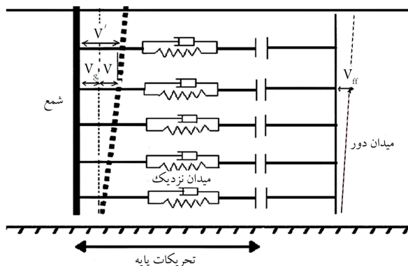
شکل ۱. مدل وینکلر جهت آنالیز دینامیکی شمع تحت اثر بار جانبی. [۲۳]
