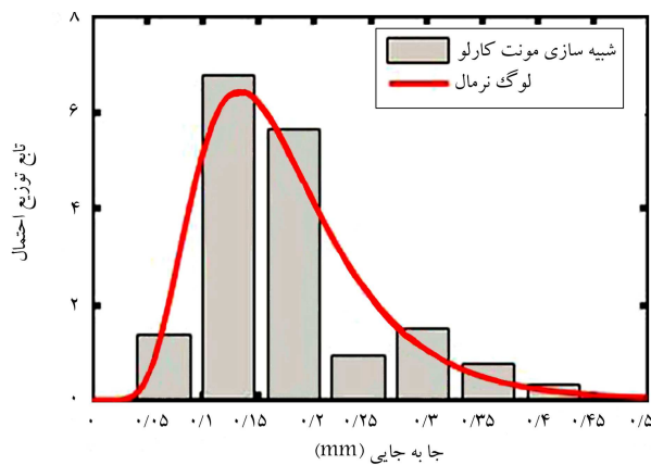
شکل ۱۶. تابع چگالی احتمال بیشینه‌ی جابه‌جایی سر شمع در ثانیه‌ی سی‌ام زلزله.
