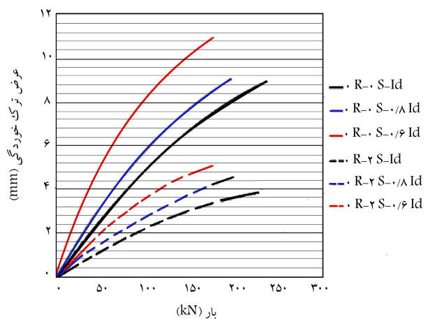
شکل ۱۹. بار متناظر با بروز ترک خوردگی در نمونه‌ی دارای سنگ‌دانه‌ی طبیعی و الیاف فولادی.
