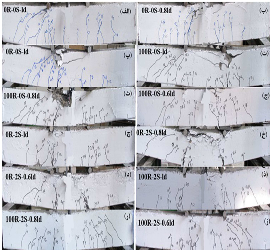
شکل ۱۴. شکست نمونه‌ها و مسیر گسترش ترک خوردگی در نمونه‌ها تحت بار استاتیکی.
