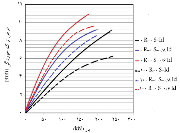
شکل ۱۷. بار متناظر با بروز ترک خوردگی در نمونه‌ی دارای سنگ‌دانه‌ی باز یافتی و طبیعی.
