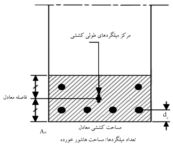
شکل ۵. تعیین مشخصات هندسی مقطع طبق آیین‌نامه‌ی ۰۱ - ACI 224R [۴۹]
