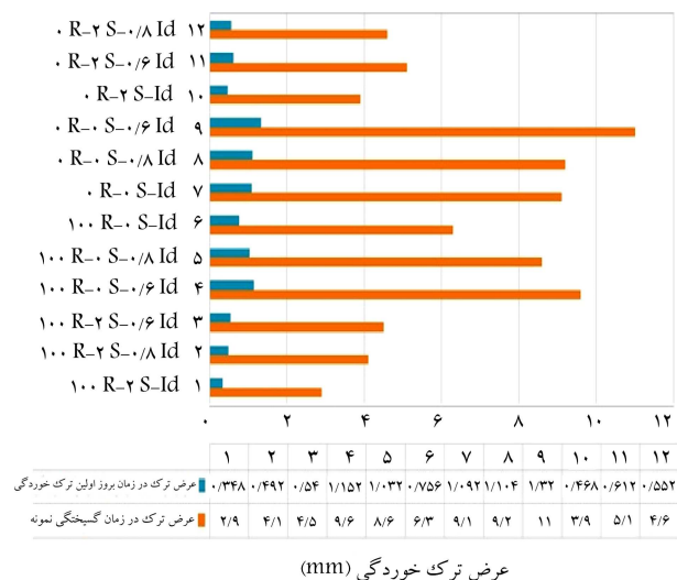
شکل ۱۵. بیشینه‌ی عرض ترک خوردگی نمونه‌ها در دو لحظه‌ی وقوع اولین ترک و شکست نمونه.
