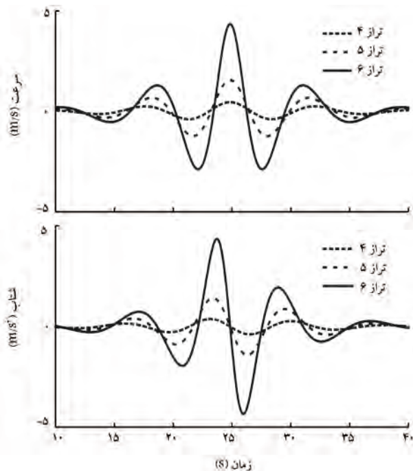
شکل ۲. سرعت و شتاب وارد بر ترازهای مختلف سکوی تحت بار موج. [۴۵]
