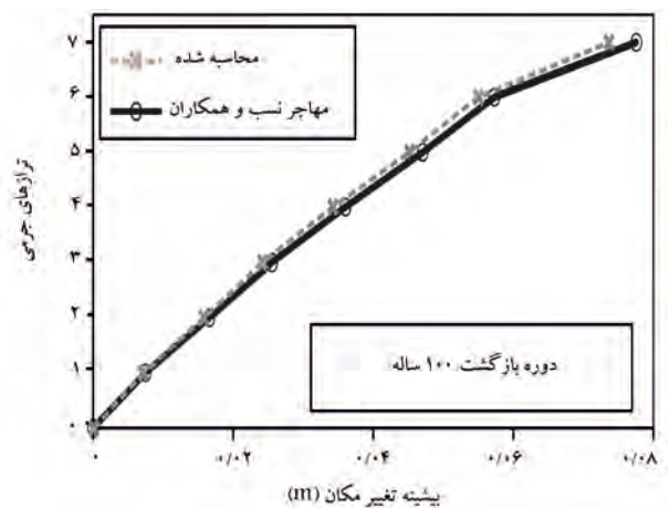
شکل ۴. مقایسه‌ی پیشینه‌ی تغییر مکان عرشه‌ی سکو تحت بارگذاری موج با دوره‌ی بازگشت ۱۰۰ سال.
