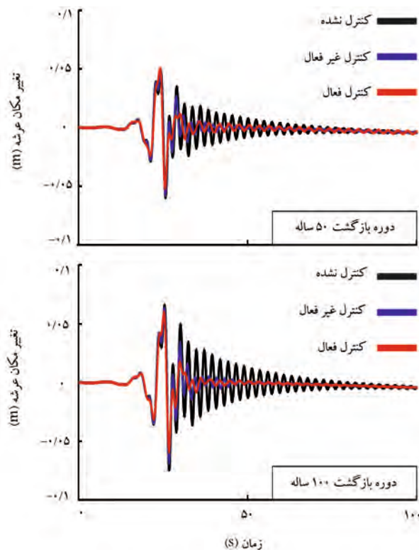
شکل ۱۰. مقایسه‌ی تاریخی‌ی زمانی جابه‌جایی عرشه.
