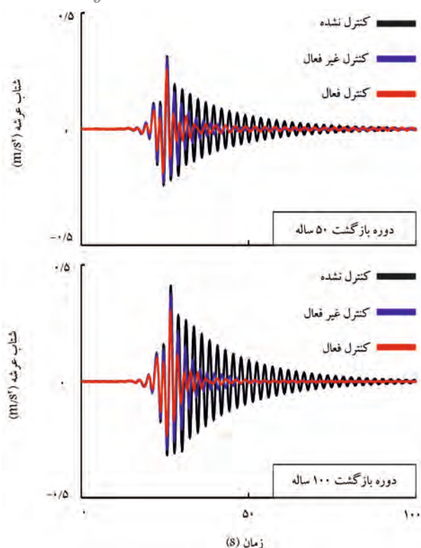
شکل ۱۱. مقایسه‌ی تاریخی‌ی زمانی شتاب عرشه.
