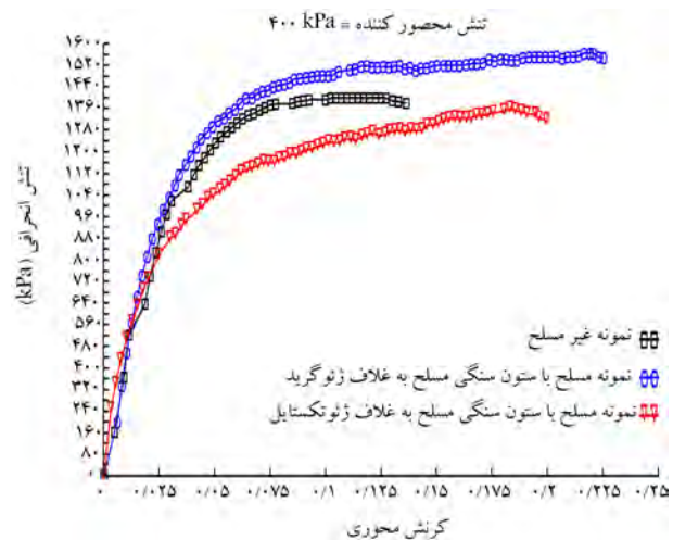
شکل ۷. نمودار تنش - کرنش در شرایط تنش محصورکننده ۴۰۰ کیلو پاسکال.
