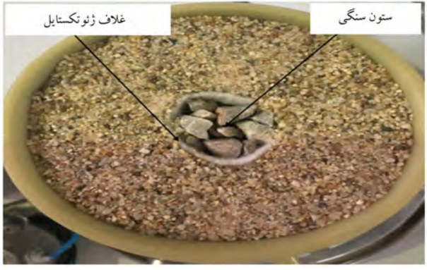
شکل ۳. ساخت ستون سنگی مسلح با غلاف ژئوتکستایل در آزمایش سه‌محوری.
