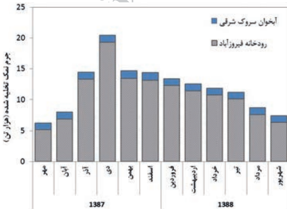
شکل ۵. جرم نمک تخلیه شده از گنبد نمکی به درون آبخوان سروک شرقی و رودخانه فیروزآباد (ارتفاع کل ستون نیز کل نمک تخلیه شده از گنبد نمکی کنارسیاه را نشان می‌دهد).
