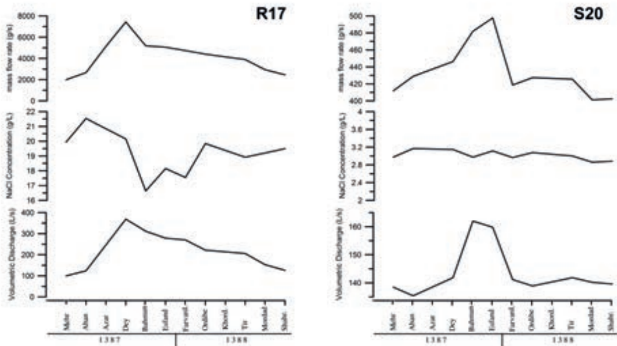
شکل ۲. هیدروگراف و کموگراف جریان پایه ایستگاه هیدرومتری R17 و چشمه کنارسياه (S20) در طول دوره نمونه‌برداری.
