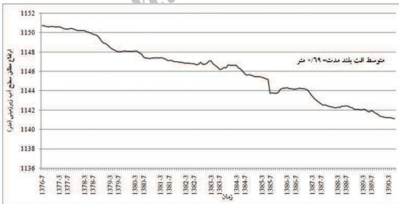
شکل ۱. هیدروگراف معرف آبخوان دشت اشتهارد در دوره ۹۰-۱۳۷۶.
