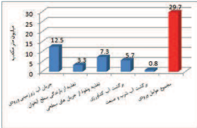
شکل ۲. عوامل ورودی و خروجی متوسط سالیانه به آبخوان دشت اشتهارد.
