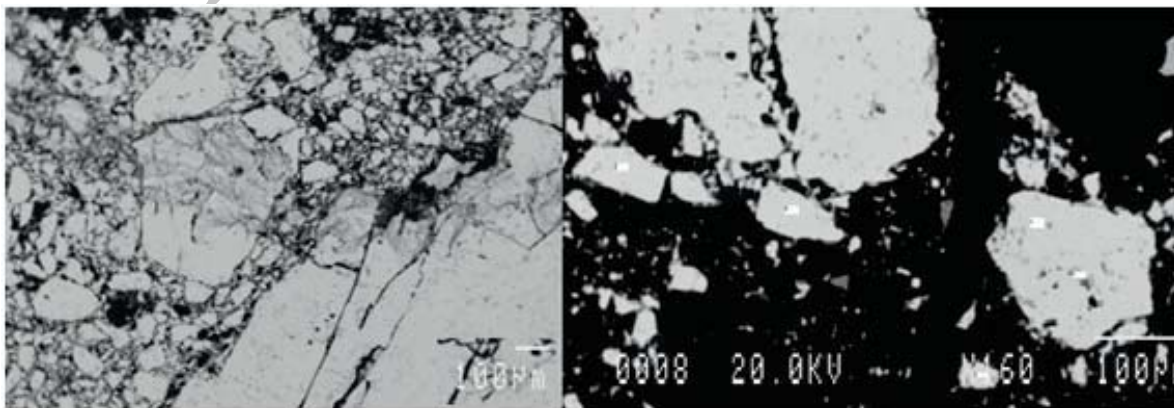
شکل ۳. تصاویر Back scattered از برشی شدن و خوردگی انحلالی اسفالریت (خاکستری) در نمونه‌های عمیق ماهور (۱۵۰ متری).
