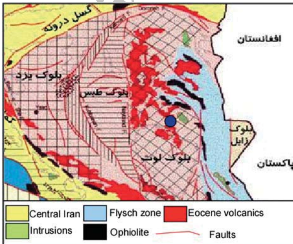
شکل ۱. موقعیت بلوک لوت نسبت به مناطق مجاور. محل تقریبی کانسارماهور با دایره آبی پرنگ مشخص شده است (آقاباتی، ۱۳۸۳؛ Stocklin 1968).
