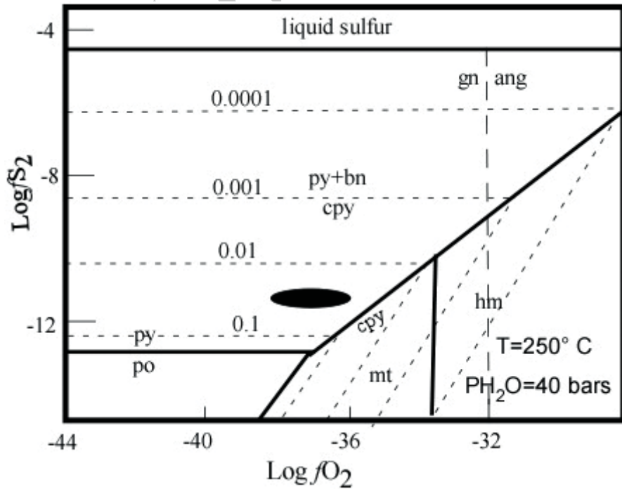
شکل ۱۰. نمودار Log fO_2 - Log fS_2 که در آن محدوده پایداری گوگرد و بعضی از سولفیدها و اکسیدها و کربنات روی مشخص شده است. خط چین‌ها مقدار آهن را در (Zn, Fe)S نشان می‌دهد. بیضی سیاه رنگ با شرایط تشکیل اسفالریت در ماهور نزدیک است.
