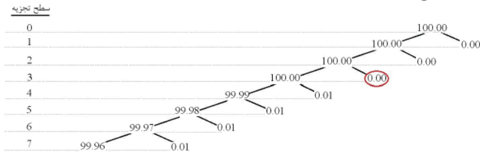
شکل ۳. تجزیه نگر چگالی چاه ۱۴-۰۹ با موجک مادر تا سطح ۷. اعداد نشان داده شده در درخت تجزیه، معرف انرژی سیگنال در هر بخش هستند. صفر شدن انرژی سیگنال در بخش جزئیات تا سطح ۳ و ناچیز بودن انرژی در بخش‌های جزئیات در سطوح بعدی مشاهده می‌شود.
