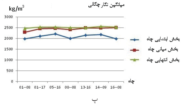
شکل ۲. خصوصیات آماری نگرها در چاه‌های مختلف میدان. الف) میانگین، معیار خوبی برای جداسازی نگر تخلص به دست آمده از چگالی در بخش ابتدایی، میانی و انتهایی چاه است، ب) انحراف معیار، نگر تخلص به دست آمده از چگالی را در بخش‌های میانی و انتهایی چاه جدا می‌سازد، پ) میانگین، نگر چگالی را تنها در بخش ابتدایی چاه جدا می‌سازد، ت) با کمک انحراف معیار سه بخش نگر چگالی در چاه‌ها از هم تفکیک می‌شوند.
