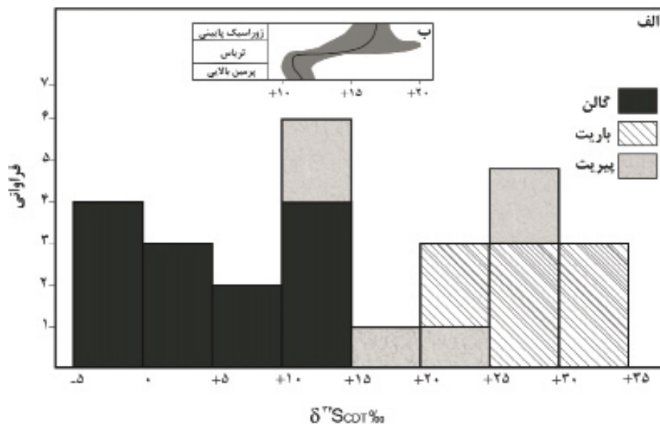
شکل ۶. توزیع ترکیب ایزوتوپی گوگرد در کانی‌های سولفیدی و سولفات کانسارهای مورد مطالعه و مقایسه آن با مقادیر \delta^{34}\text{S} سولفات آب دریای تریاس (منحنی ترکیب ایزوتوپی گوگرد سولفات آب دریا مربوط به پرمین پایانی- تریاس- ژوراسیک آغازین از Claypool et al., 1980).
