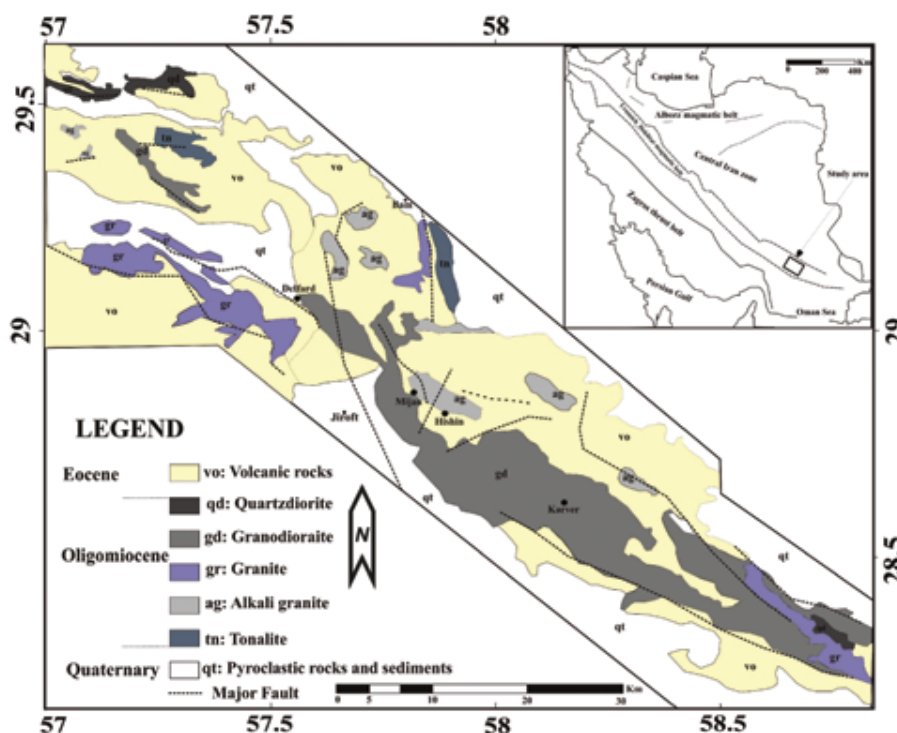
شکل ۱. نقشه زمین‌شناسی مجموعه گرانیتوئیدی جبال بارز (اقتباس از نقشه‌های زمین‌شناسی ۱:۱۰۰۰۰۰ سبزواری، نورماشیر و بزم)
