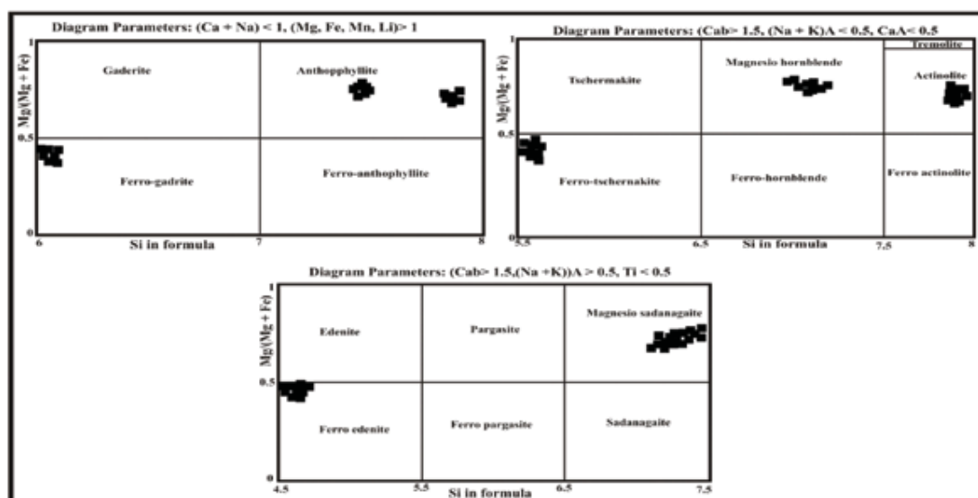
شکل ۴. تقسیم‌بندی آمفیبول‌های منطقه جبال بارز بر اساس روش Laeke (1997)
