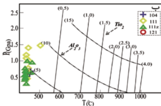
شکل ۶. الف) محدوده‌ی دمایی بیوتیت‌های منطقه حلب - میانج در فشار ثابت (Henry and Guidotti, 2005) 4/6 Kbar، ب) نمودار دما-فشار و ایزوپلیت‌های اکسیدهای اصلی \text{TiO}_2 و \text{Al}_2\text{O}_3 در آمفیبول‌های مقطع حلب - میانج (Ernst and Liu, 1998)
