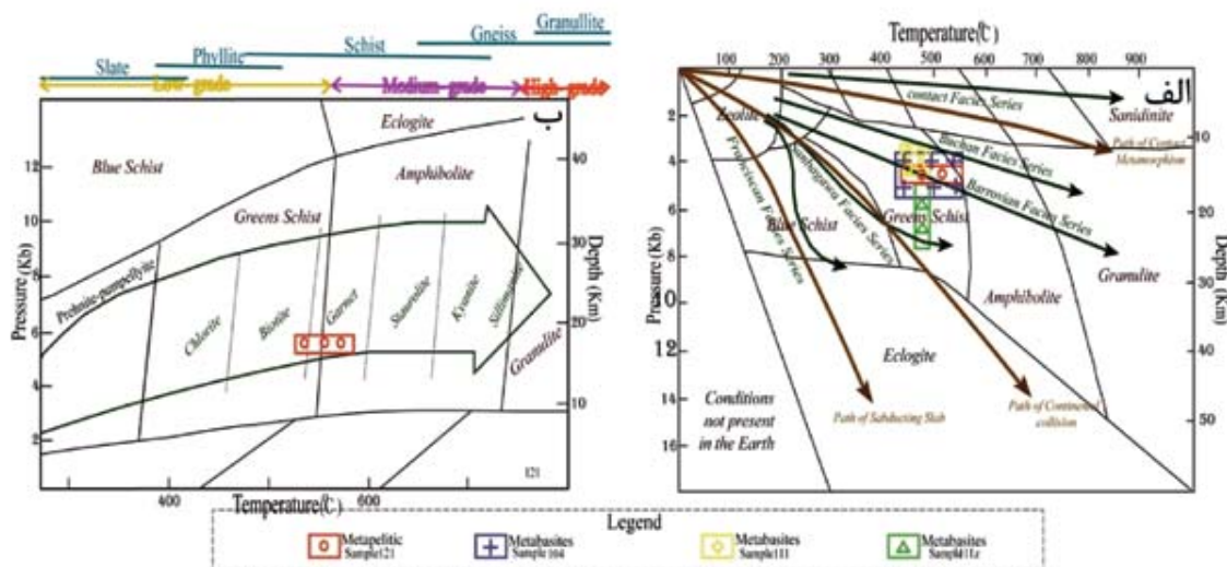
شکل ۷. الف) نمودار دما- فشار و مناطق پایداری نمونه‌های مورد بررسی از لحاظ رخساره‌های دگرگونی، سری رخساره‌ها و جایگاه‌های تکتونیکی (Yardly, 1989)، ب) محدوده دما- فشار و رخساره‌ها، زون‌های دگرگونی و ساخت‌های احتمالی نمونه‌های متاپلیتی مقطع حلب - میانج با استفاده از نتایج ترموبارومتري (Miyashiro, 1973؛ Yardly, 1989)
