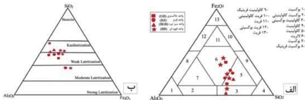
شکل ۳. الف) نمودار سه‌تایی \text{Al}_2\text{O}_3\text{-Fe}_2\text{O}_3\text{-SiO}_2 (Alleva, 1994) برای تعیین نوع رخساره، ب) نمودار سه‌تایی \text{SiO}_2\text{-Fe}_2\text{O}_3\text{-Al}_2\text{O}_3 (Schellmann, 1986) برای تعیین نوع هوازدگی در نهشته شیرین‌آباد
