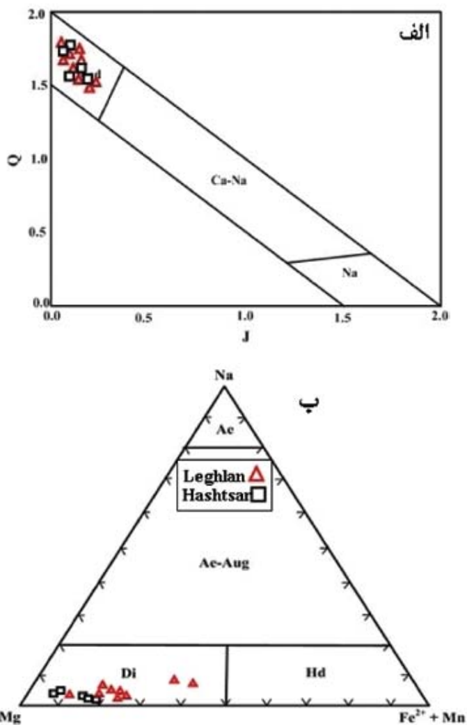
شکل ۵. الف) جدایش پیروکسن های کلسیک، کلسیک-سدیک و سدیک بر پایه نمودار (Q-J، Morimoto et al., 1988)، ب) ترکیب شیمیایی کلینوپیروکسن های موجود در گابروهای منطقه بر روی نمودار مثلثی (Mg-Na-(Fe 2+ +Mn)، Eby et al., 1998).
