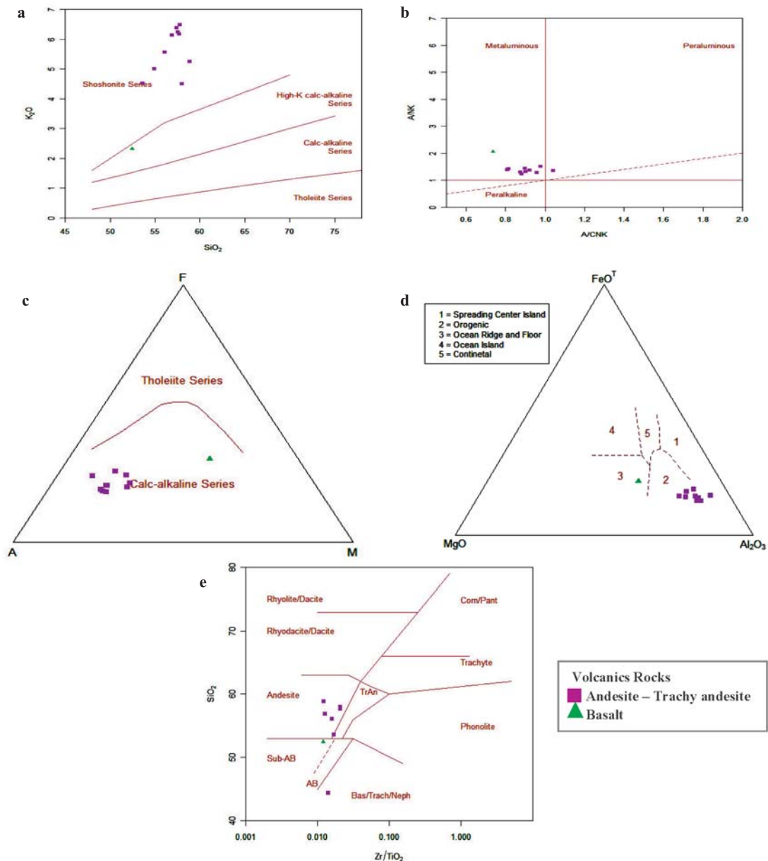
شکل ۹. (a) نمودار تعیین شاخص پتاسیم (Peccerillo and Taylor, 1976)؛ (b) نمودار تعیین شاخص آلومینیوم (Shand, 1943)؛ (c) نمودار جهت تفکیک سنگ‌های آذرین کالک آلکالین از تولیتی؛ (d) نمودار جداکننده محیط‌های تکتونیکی سنگ‌های آتشفشانی؛ (e) نمودار مقدار اکسید سیلیسیم به نسبت زیرکن به اکسید تیتانیوم (Winchester and Floyd, 1977)
