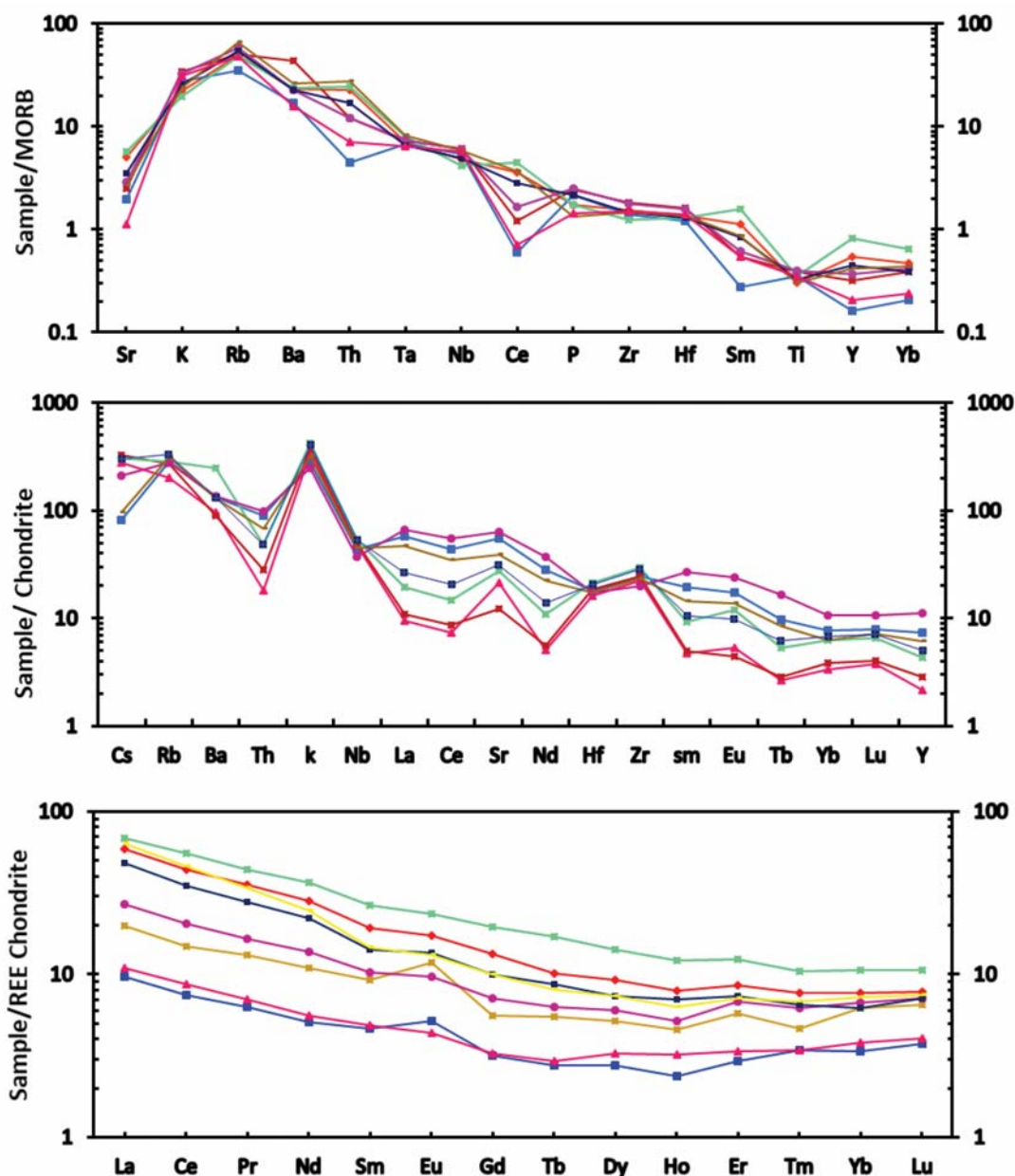
شکل ۱۰. (a) نمودار عنکبوتی سنگ‌های آتشفشانی نرمالایزه شده نسبت به MORB در منطقه گل‌چشمه، بر اساس مقادیر استاندارد (Pearce, 1983) (b) نمودار عنکبوتی سنگ‌های آتشفشانی نرمالایزه شده نسبت به کندریت در منطقه گل‌چشمه، بر اساس مقادیر استاندارد (Gerlach, 1988) (c) نمودار عنکبوتی سنگ‌های آتشفشانی نرمالایزه شده نسبت به کندریت در منطقه گل‌چشمه، بر اساس مقادیر استاندارد (Boynton, 1984)
