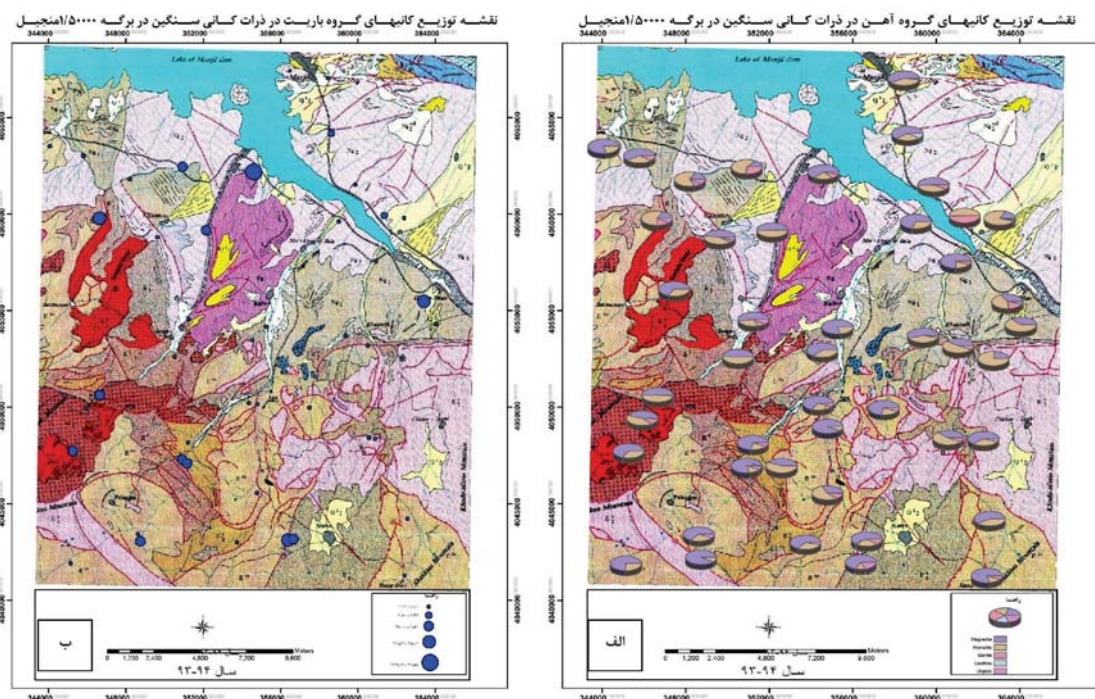
شکل ۴. الف) نقشه توزیع کانهای گروه آهن در ذرات کانی سنگین در برگه ۱:۵۰۰۰۰/منجیل، ب) نقشه توزیع کانهای گروه باریت در ذرات کانی سنگین در برگه ۱:۵۰۰۰۰/منجیل مورد مطالعه
