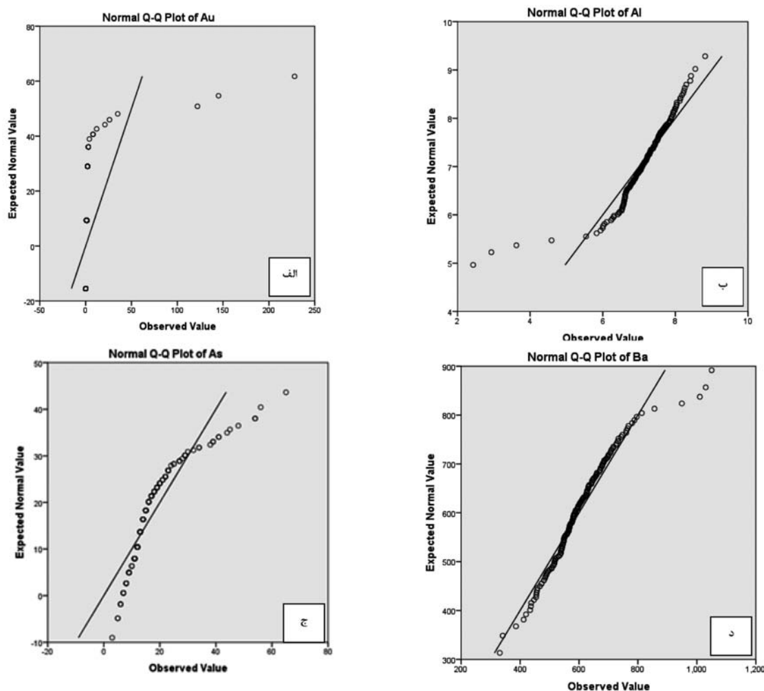
شکل ۷. نمودارهای Q-QPlot؛ الف) نمودار Q-QPlot برای عنصر طلا، ب) نمودار Q-QPlot برای عنصر آلومینیوم، ج) نمودار Q-QPlot برای عنصر آرسنیک، د) نمودار Q-QPlot برای عنصر باریم
