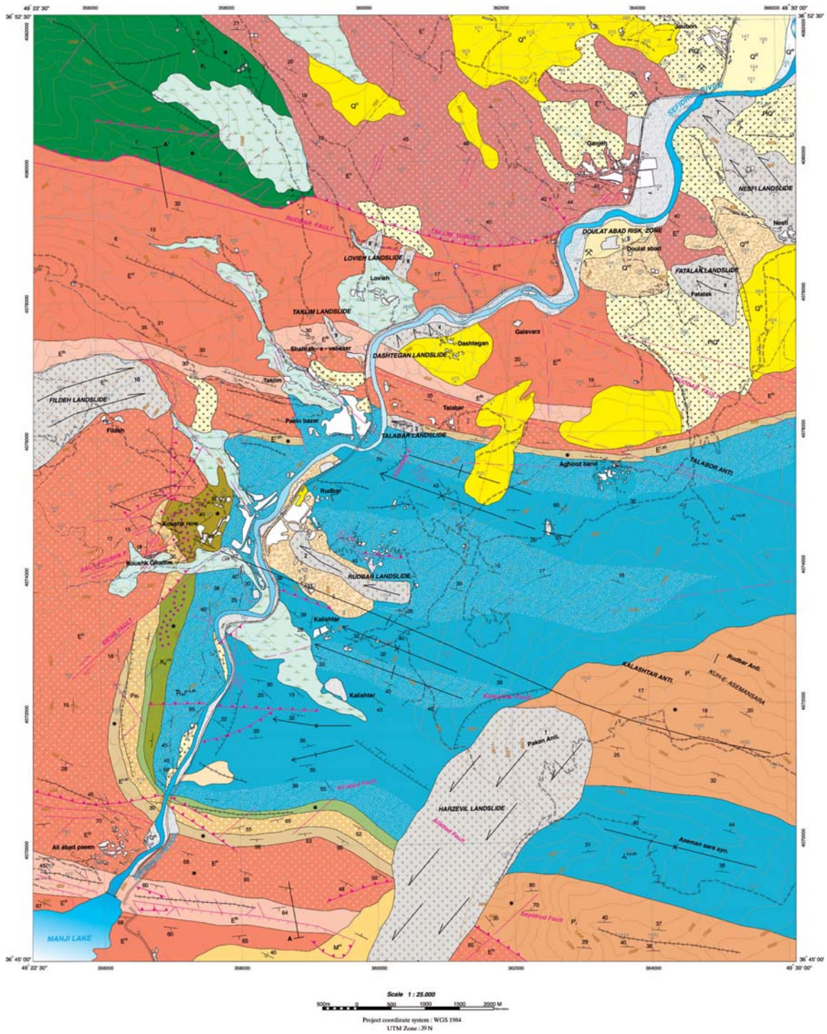
شکل ۲. نقشه زمین‌شناسی منطقه مورد مطالعه (سازمان زمین‌شناسی و اکتشافات معدنی کشور، ۱۳۸۷)
